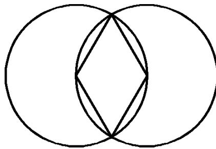
FIG. 1.—THE VESICA PISCIS
