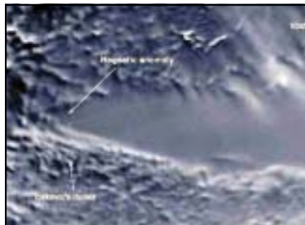
Lake Vostok's magnetic anomaly region (NASA)
