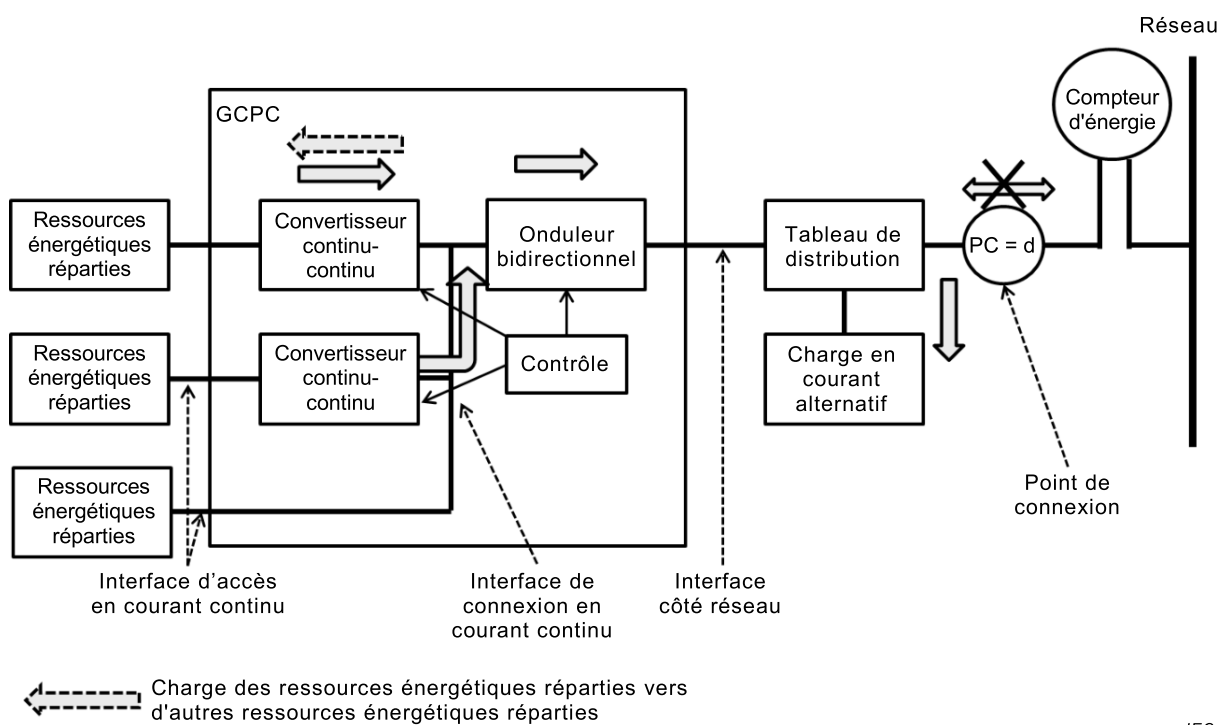
Figure 4 – Flux d'alimentation de mode III
