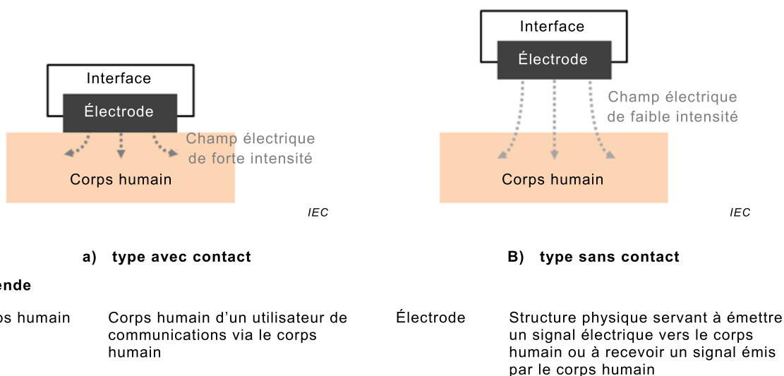
Figure 1 – Interfaces pour les communications via le corps humain
