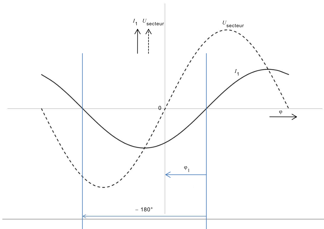
Figure E.2 – Définition de l'angle de déphasage du courant fondamental \phi_1 ( I_1 est en retard par rapport à U_{mains} , \phi_1 < 0 )
