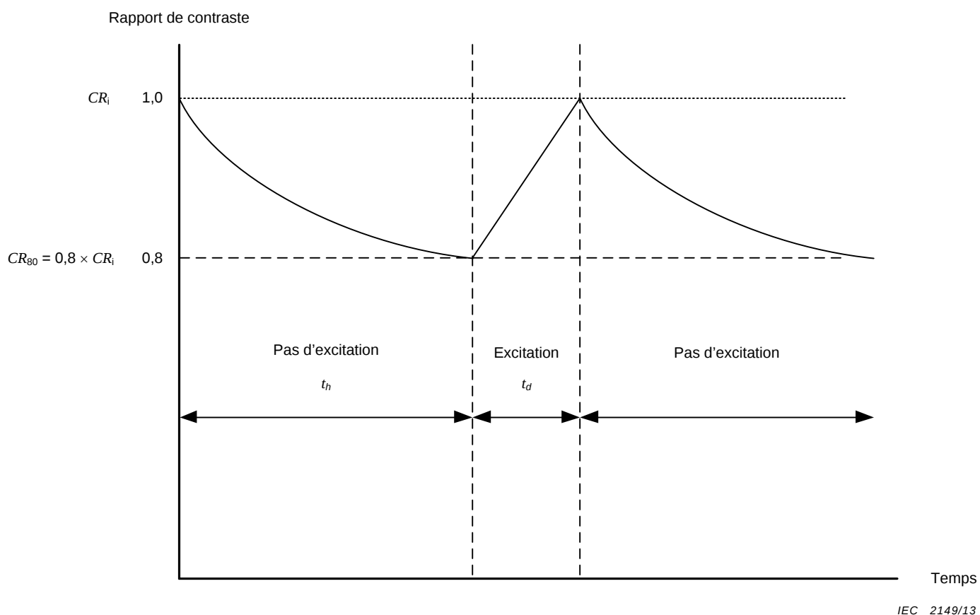
Figure 11 – Contraste d'image et mode d'excitation
