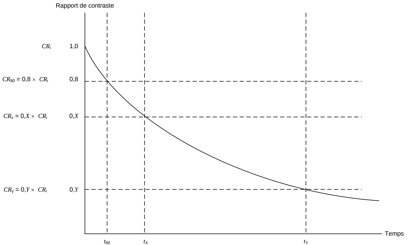
Figure 10 – Caractéristique temporelle du rapport de contraste
