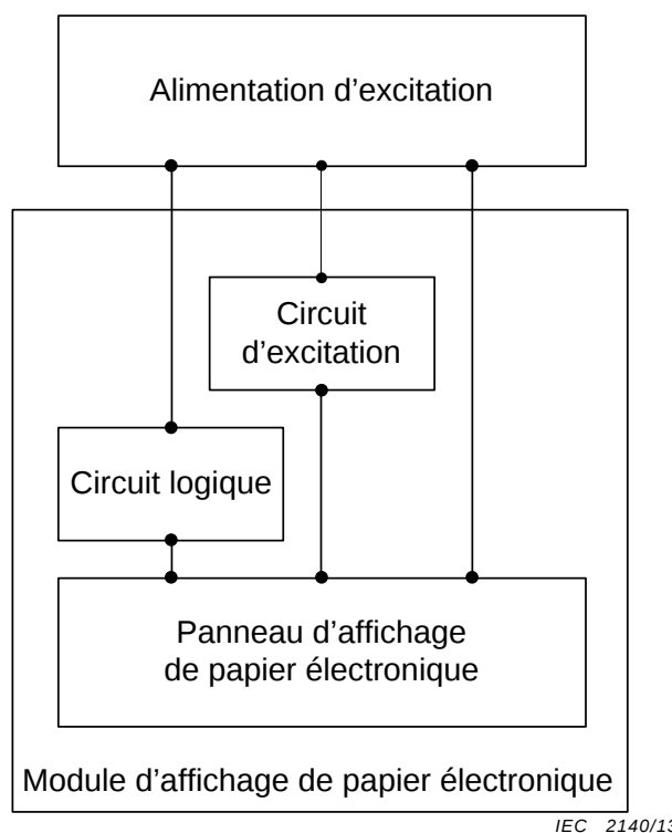
Figure 4 – Exemple de schéma fonctionnel de panneau et de module d'affichage de papier électronique
