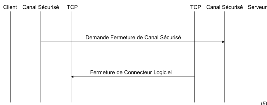
Figure 16 – Fermeture d’une connexion OPC UA TCP
