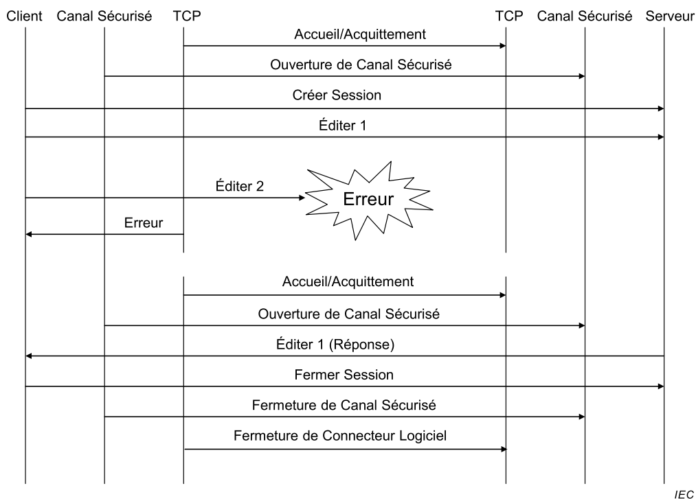
Figure 17 – Rétablissement d'une connexion OPC UA TCP
