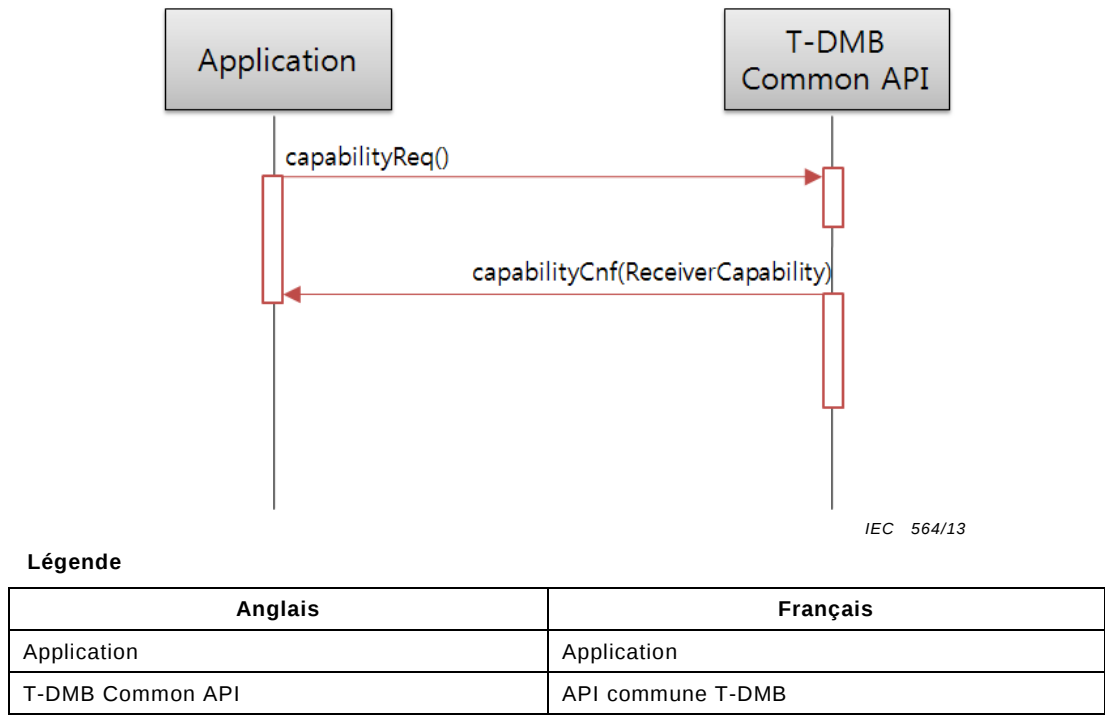
Figure 3 – Obtention des capacités du récepteur
