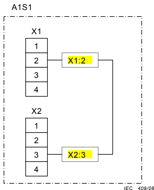
Figure 3 – Exemple d'étiquetage du raccordement de terminaison locale
