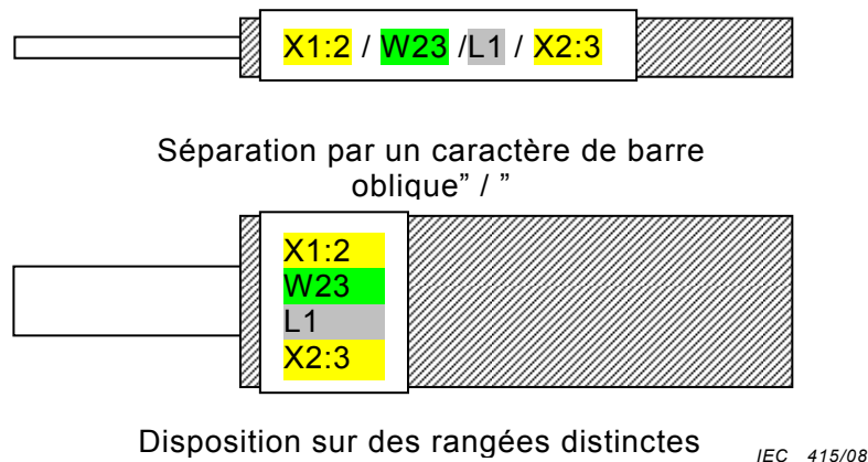
Figure 9 – Exemples de dispositions d'étiquetage sur des conducteurs isolés ou des câbles.
