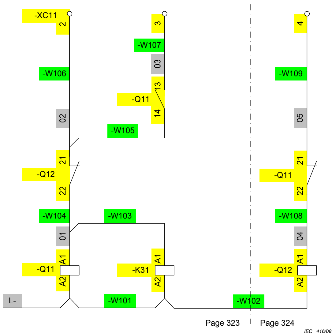
Figure A.1 – Schéma des circuits utilisé comme base pour les exemples
