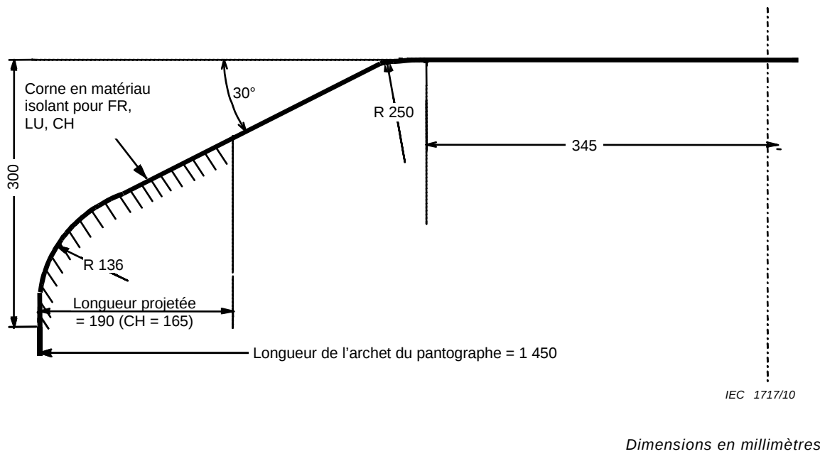
Figure B.2 – Archet du pantographe d'une longueur de 1 450 mm
