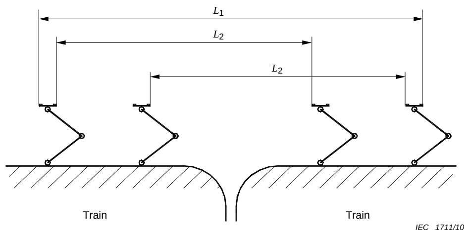
Figure A.6 – Disposition des pantographes sur les trains
