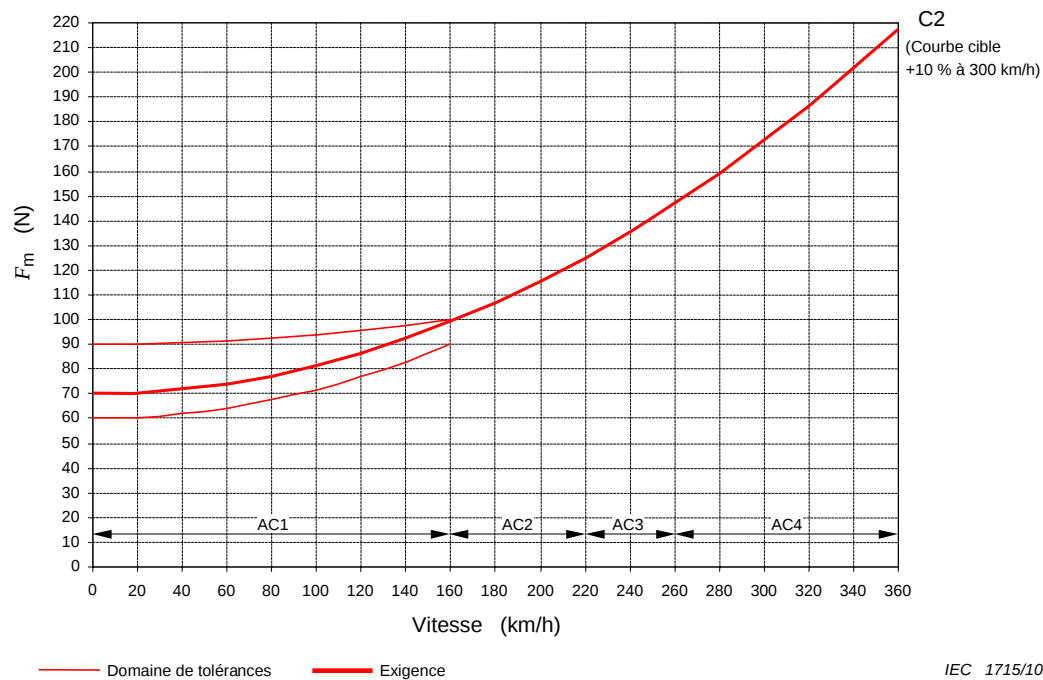
Figure B.1a – Force moyenne de contact F_m (+ 10 %) en fonction des vitesses de circulation pour FR (voir Tableau B.5)
