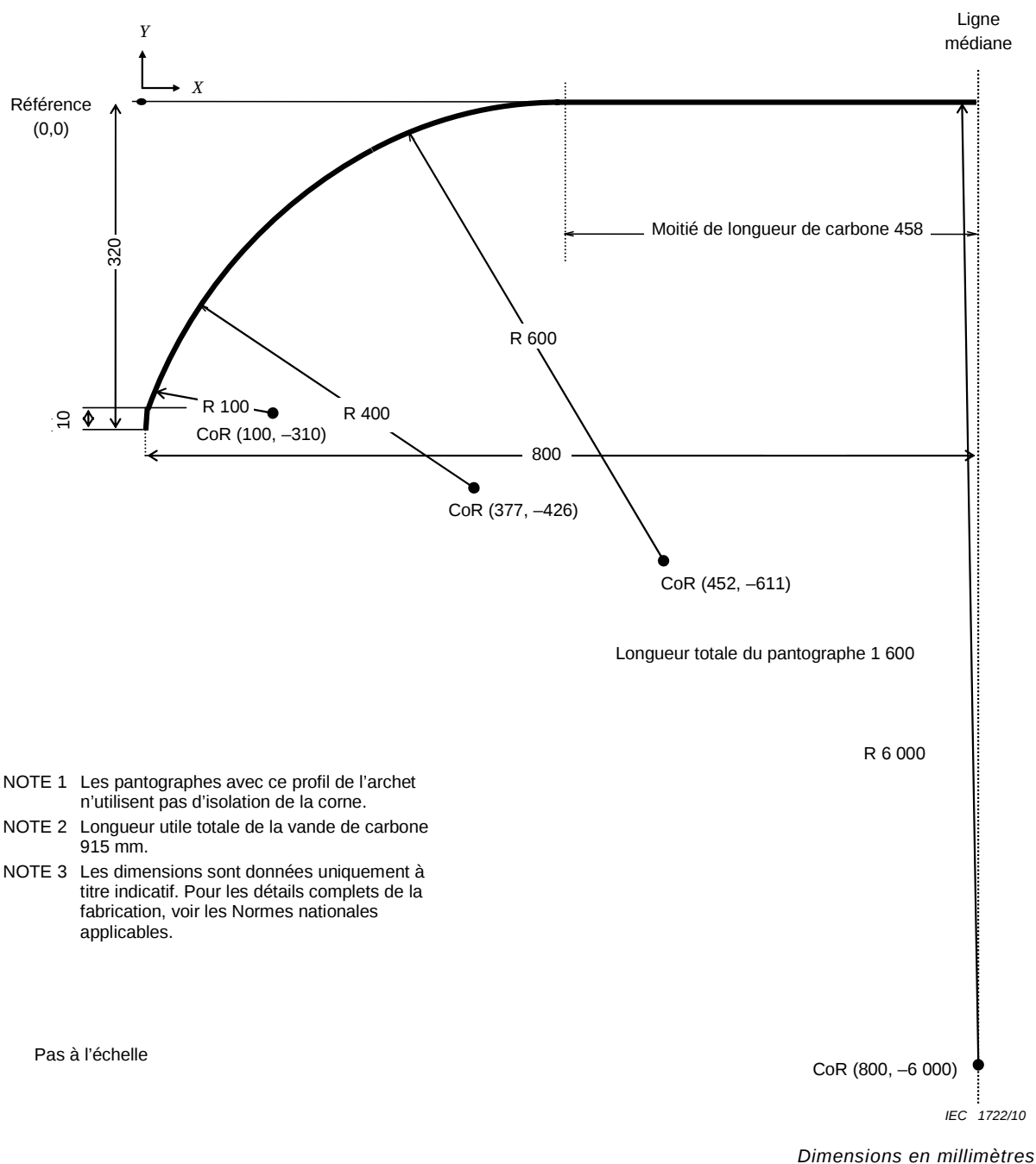
Figure B.7 – Archet du pantographe avec une longueur de 1 600 mm (GB)
