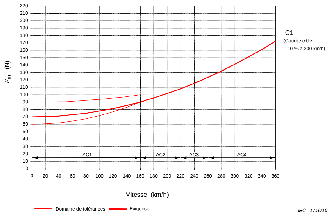
Figure B.1b – Force moyenne de contact F_m (-10 %) en fonction des vitesses de circulation pour CH, DE (voir Tableau B.5)
