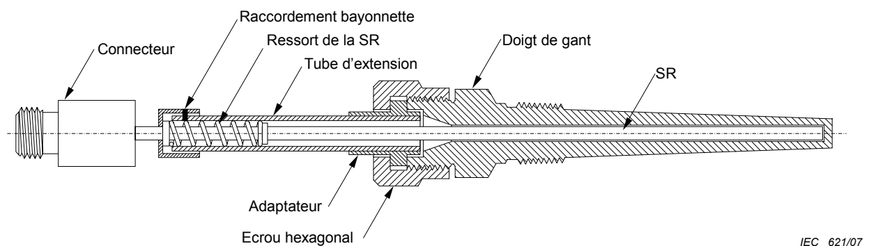
Figure 1 – Forme et dimensions d'une SR
