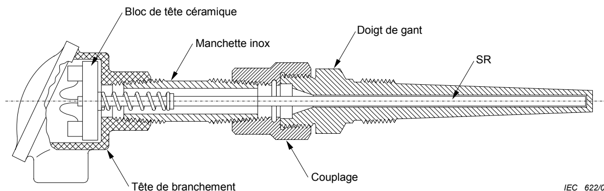
Figure 3 – Installation d'une SR rigide (Type II) à insertion longue
