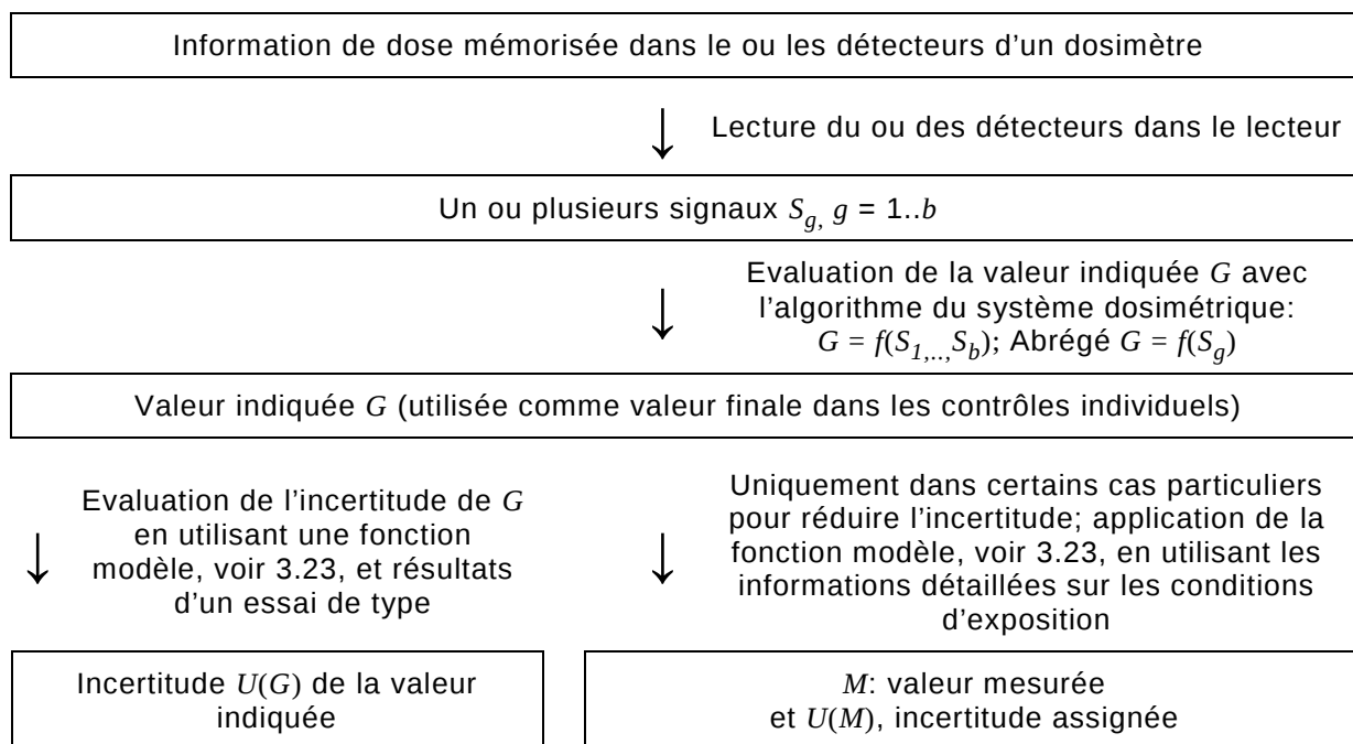
Figure B.1 – Evaluation des données d'un système dosimétrique
