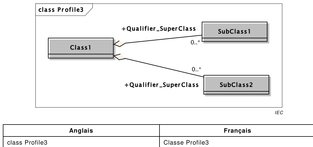
Figure C.10 – Nom de rôle d'extrémité avec qualificatif dans le modèle contextuel
