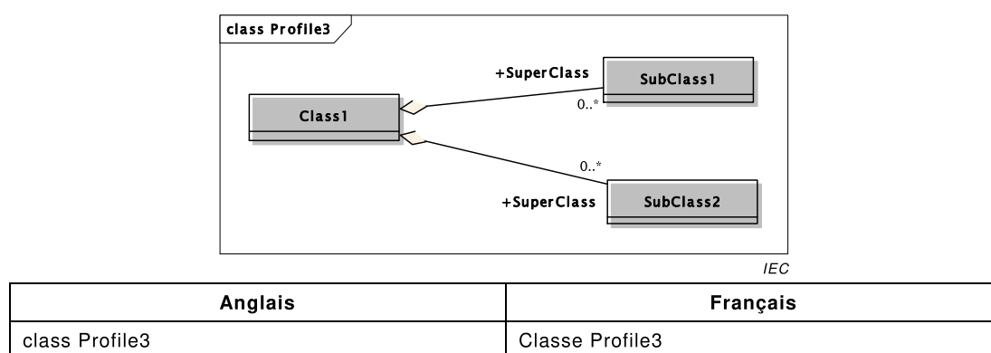
Figure C.8 – Nom de rôle d'extrémité dans le modèle contextuel coïncidant avec le nom de la superclasse
