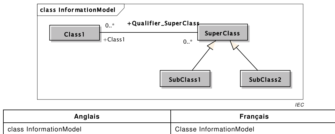
Figure C.9 – Exemple de nom de rôle d'extrémité avec qualificatif
