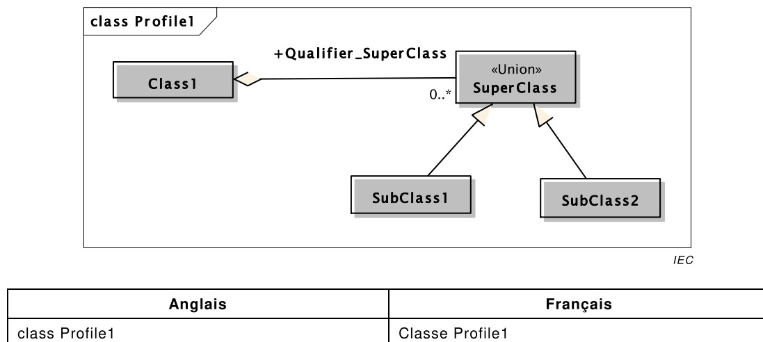
Figure C.4 – Nom de rôle d'extrémité avec qualificatif dans le modèle contextuel
