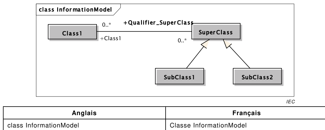
Figure C.3 – Exemple de nom de rôle d'extrémité avec qualificatif
