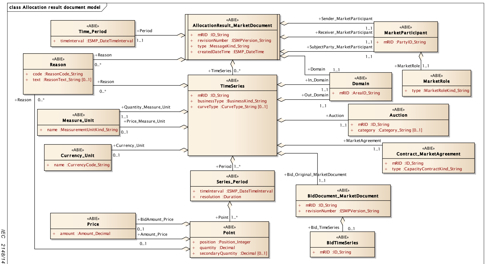
Figure 15 – Modèle contextuel de résultat de l'attribution
