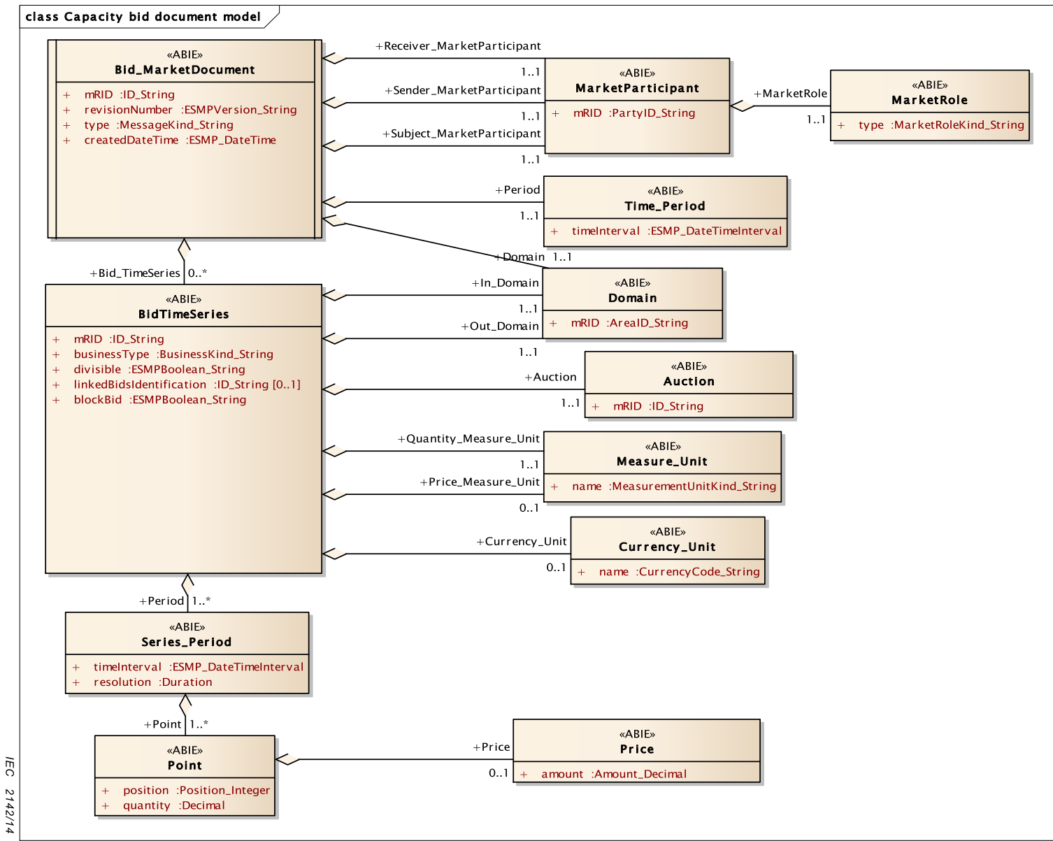
Figure 9 – Modèle contextuel d'offre
