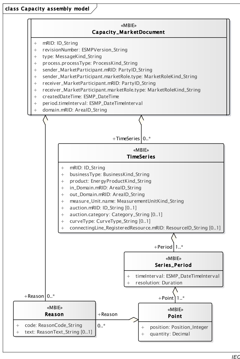
Figure 14 – Modèle d'assemblage de capacité
