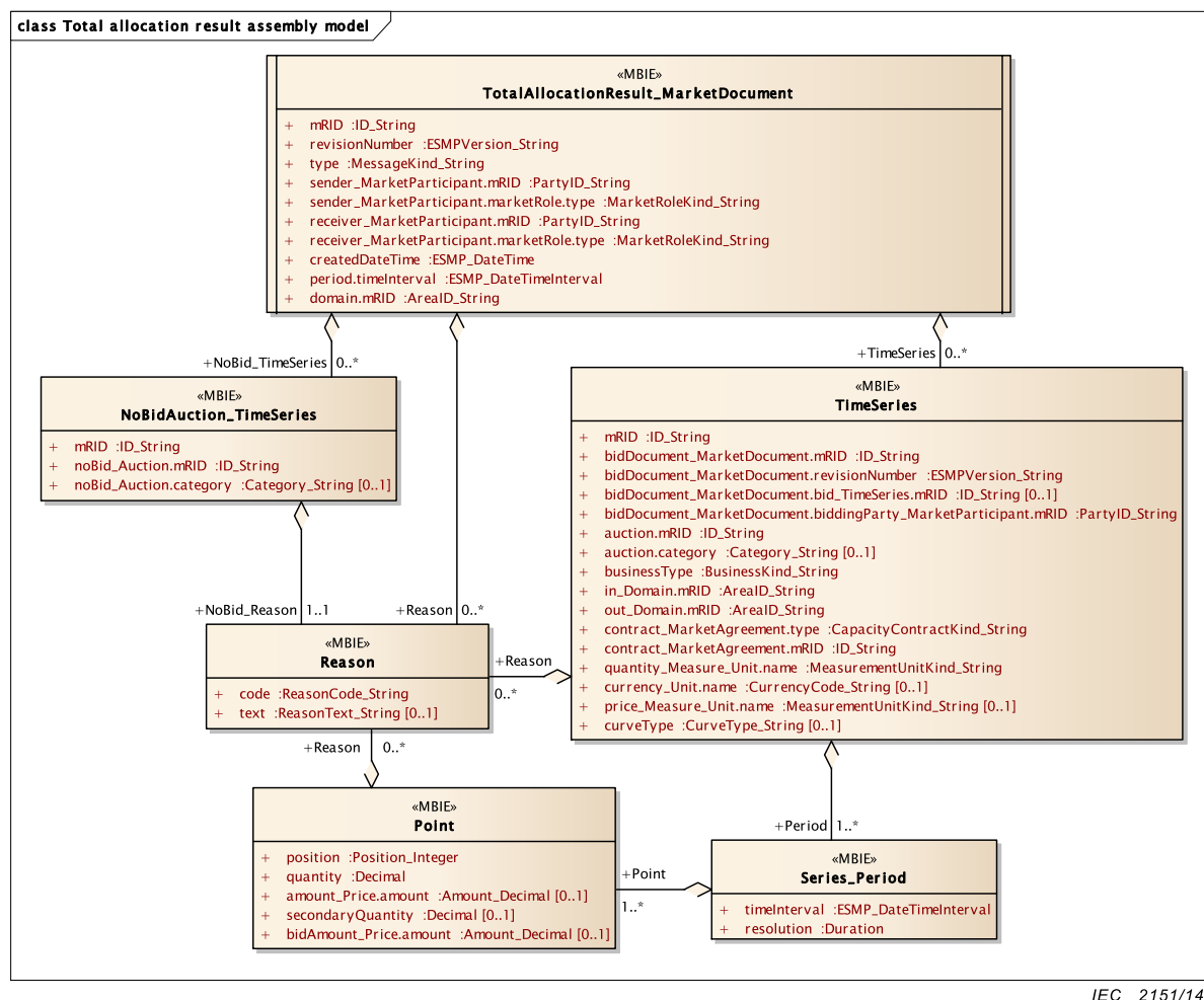
Figure 18 – Modèle d'assemblage de résultat de l'attribution totale
