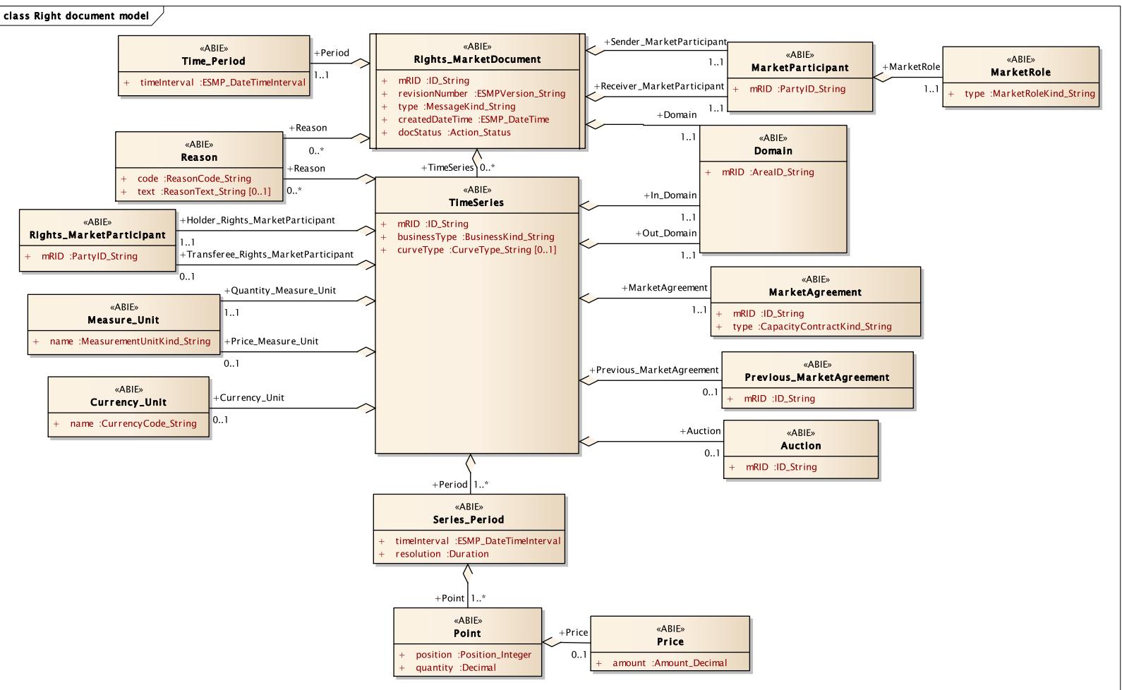
Figure 23 – Modèle contextuel des droits
