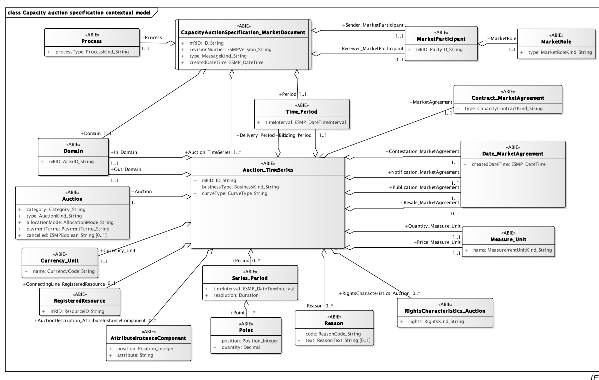
Figure 11 – Modèle contextuel de spécification de vente aux enchères de capacité
