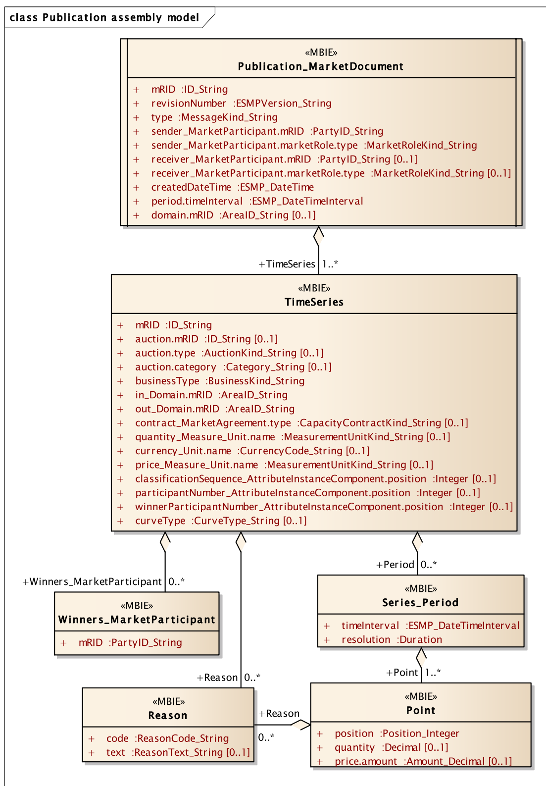
Figure 22 – Modèle d'assemblage de publication
