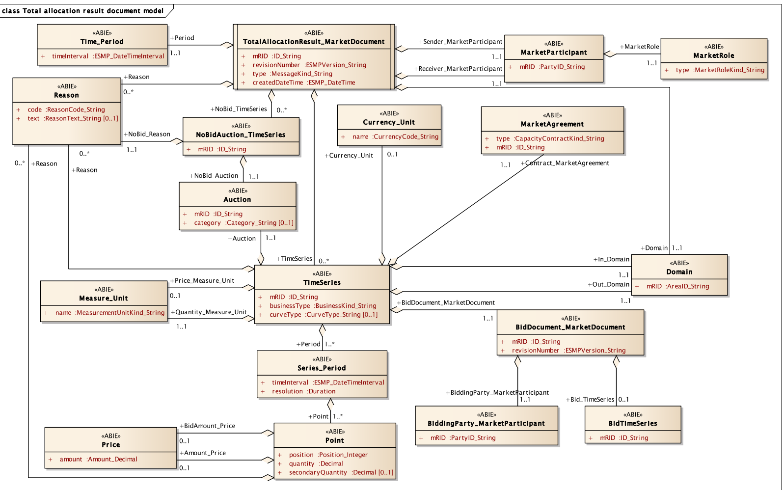
Figure 17 – Modèle contextuel de résultat de l'attribution totale
