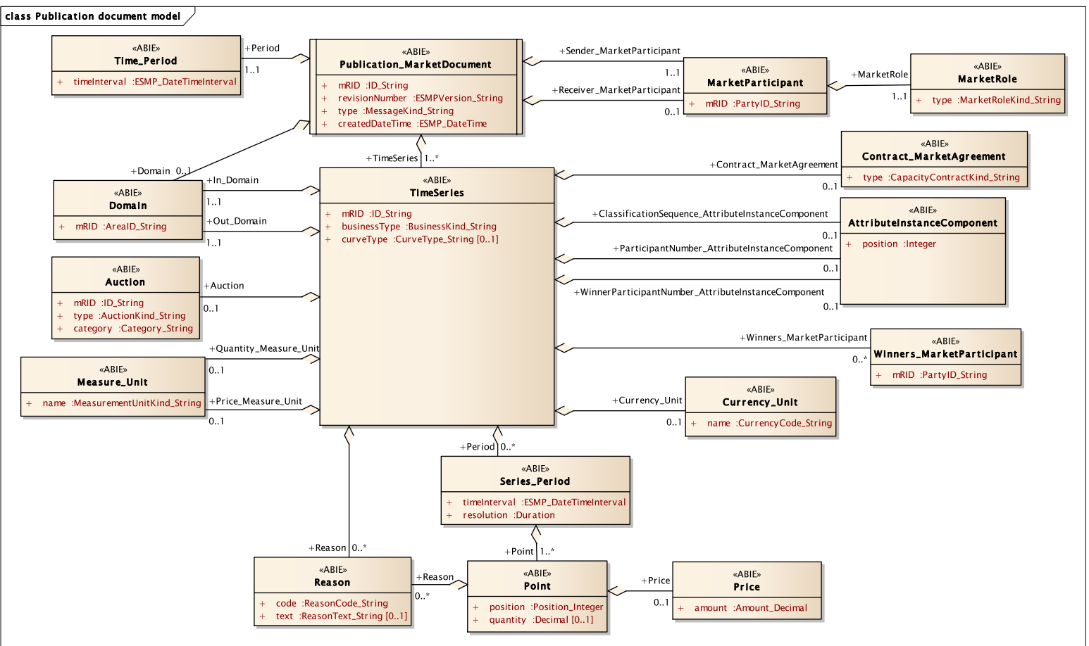
Figure 21 – Modèle contextuel de publication
