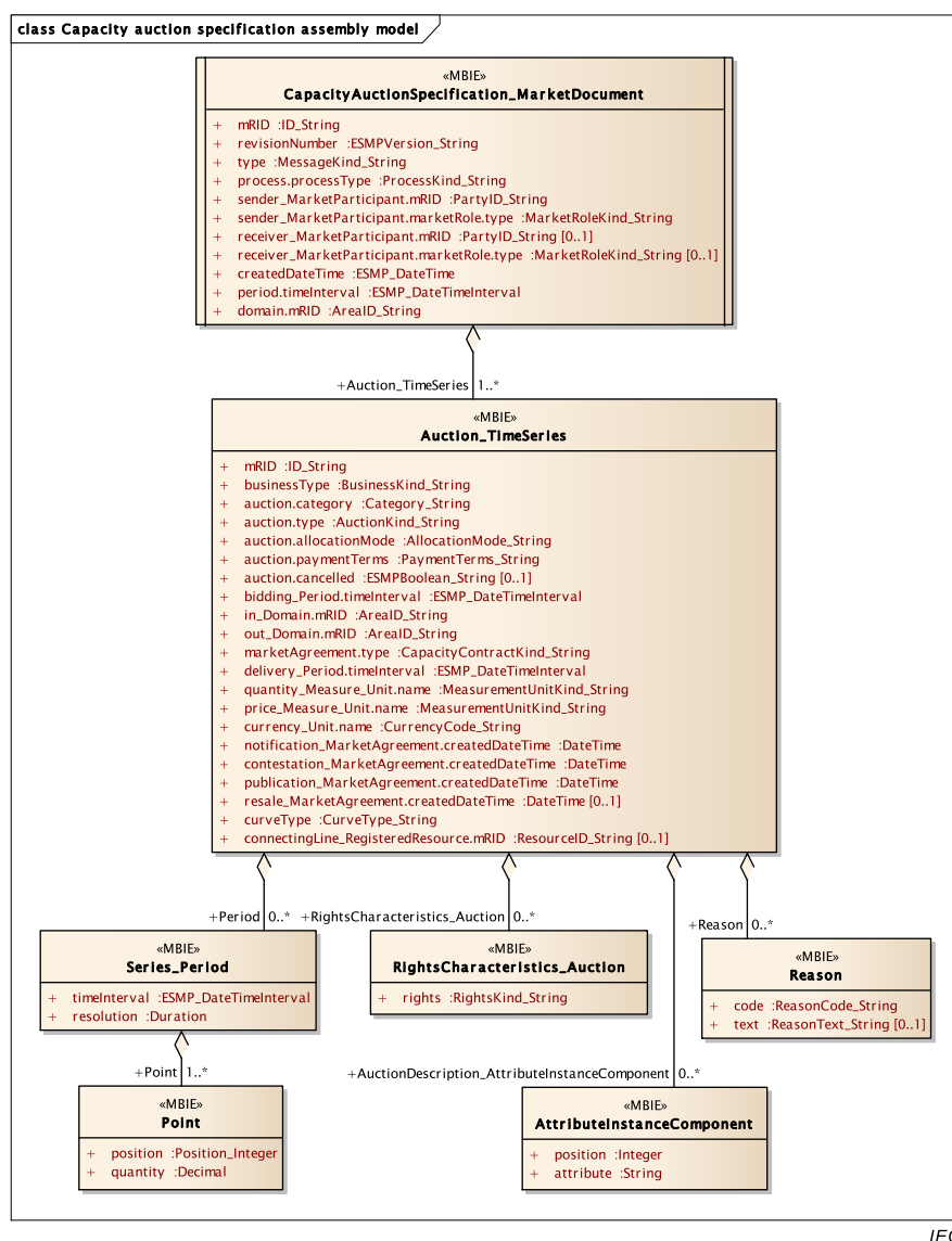
Figure 12 – Modèle d’assemblage de spécification de vente aux enchères de capacité
