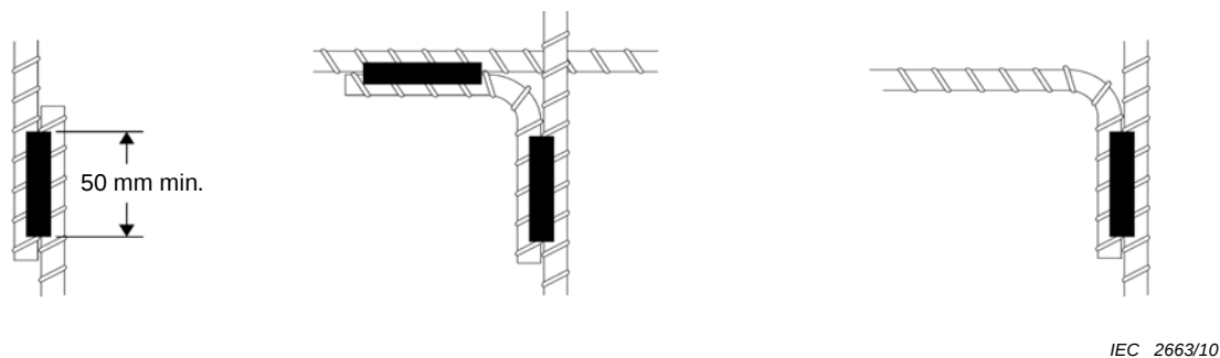
Figure E.5a - Jonctions soudées (adaptées au courant de foudre et à la CEM)
