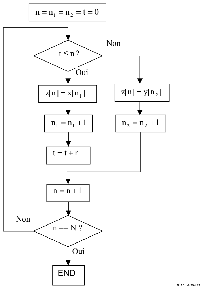
Figure 9 – Organigramme de la méthode d'entrelacement
