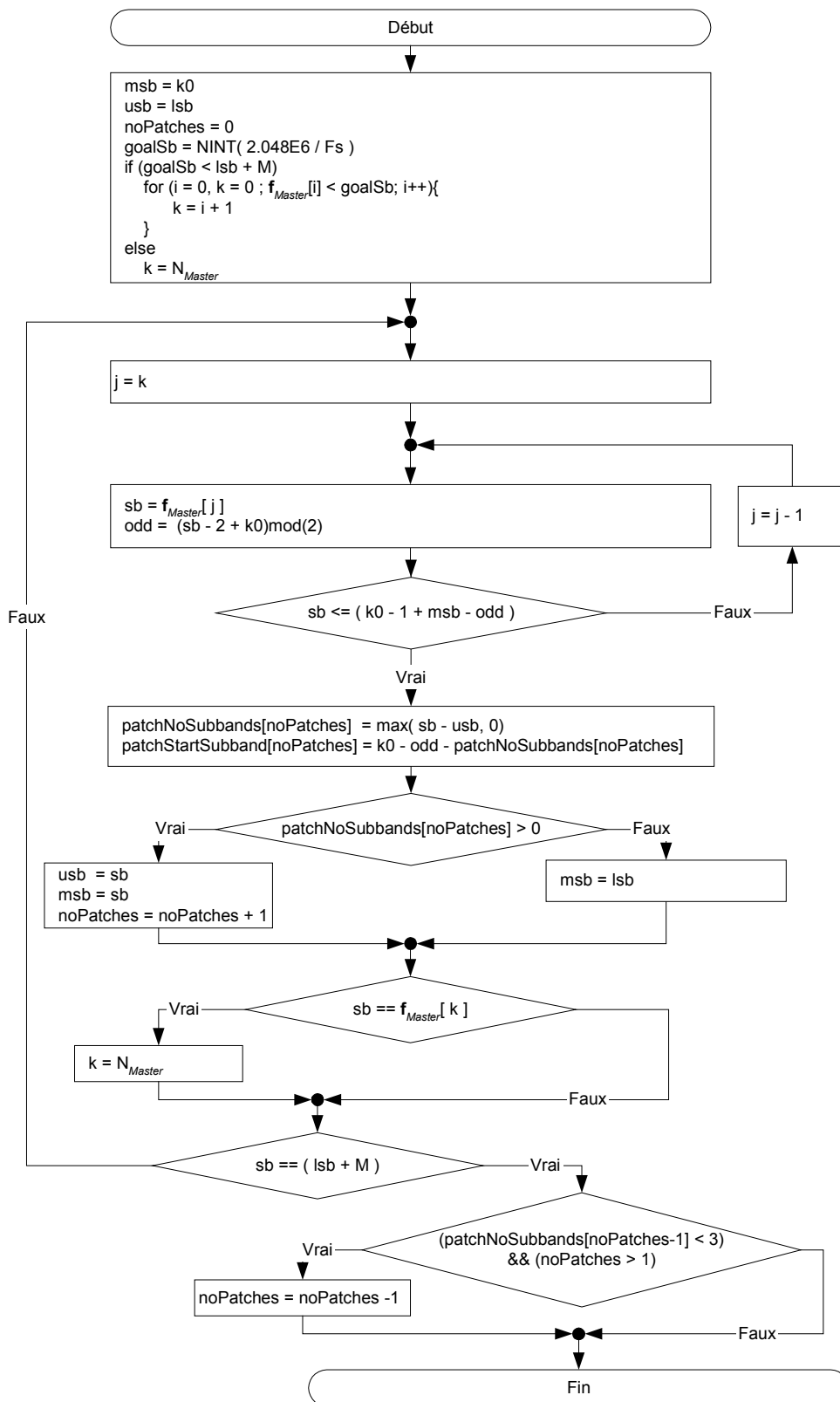
Figure 17 – Organigramme de réalisation de la transposition
