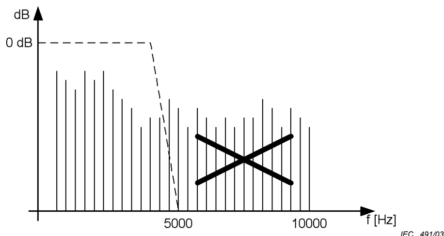
Figure 12 – Exemple de limitation de bande pour un signal typique
