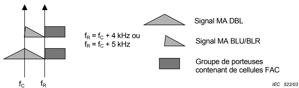
Figure K.2 – Exemple de modes simulcast avec un décalage d'un demi-canal
