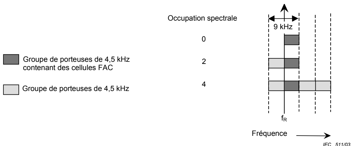
Figure 32 – Occupation spectrale dans le cas des canaux à 9 kHz
