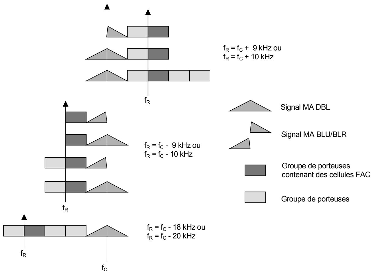
Figure K.1 – Exemple de modes simulcast avec un décalage d'un nombre entier de canaux
