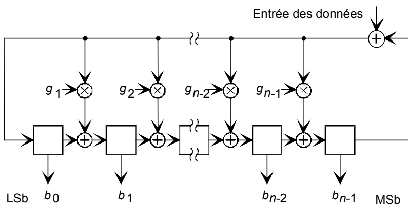
Figure D.1 – Schéma synoptique général du CRC
