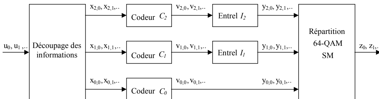
Figure 21 – Codage multi-niveaux à 3 niveaux pour SM
