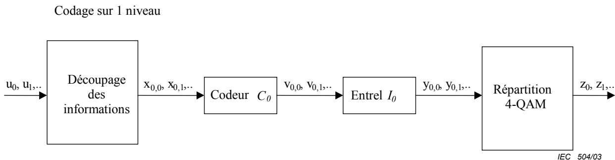
Figure 25 – Codage multi-niveaux à 1 niveau (SM)
