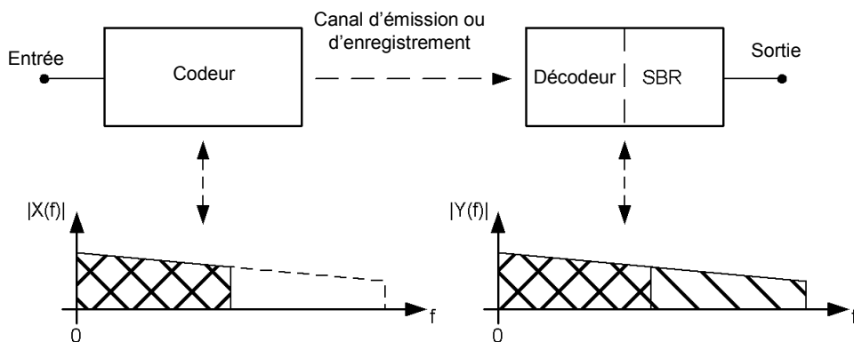
Figure 11 – Le système de codage de source avec SBR
