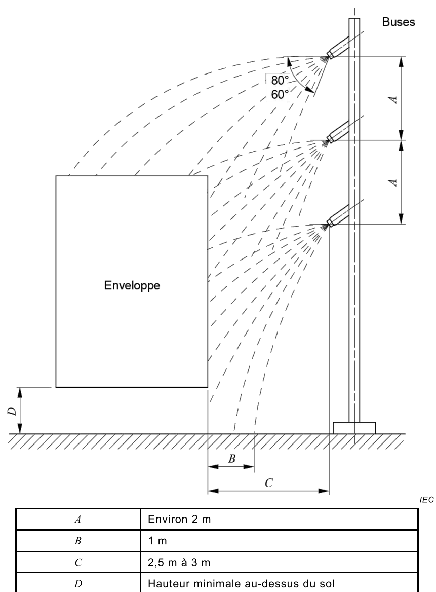
Figure C.1 – Disposition pour l'essai de protection contre les intempéries
