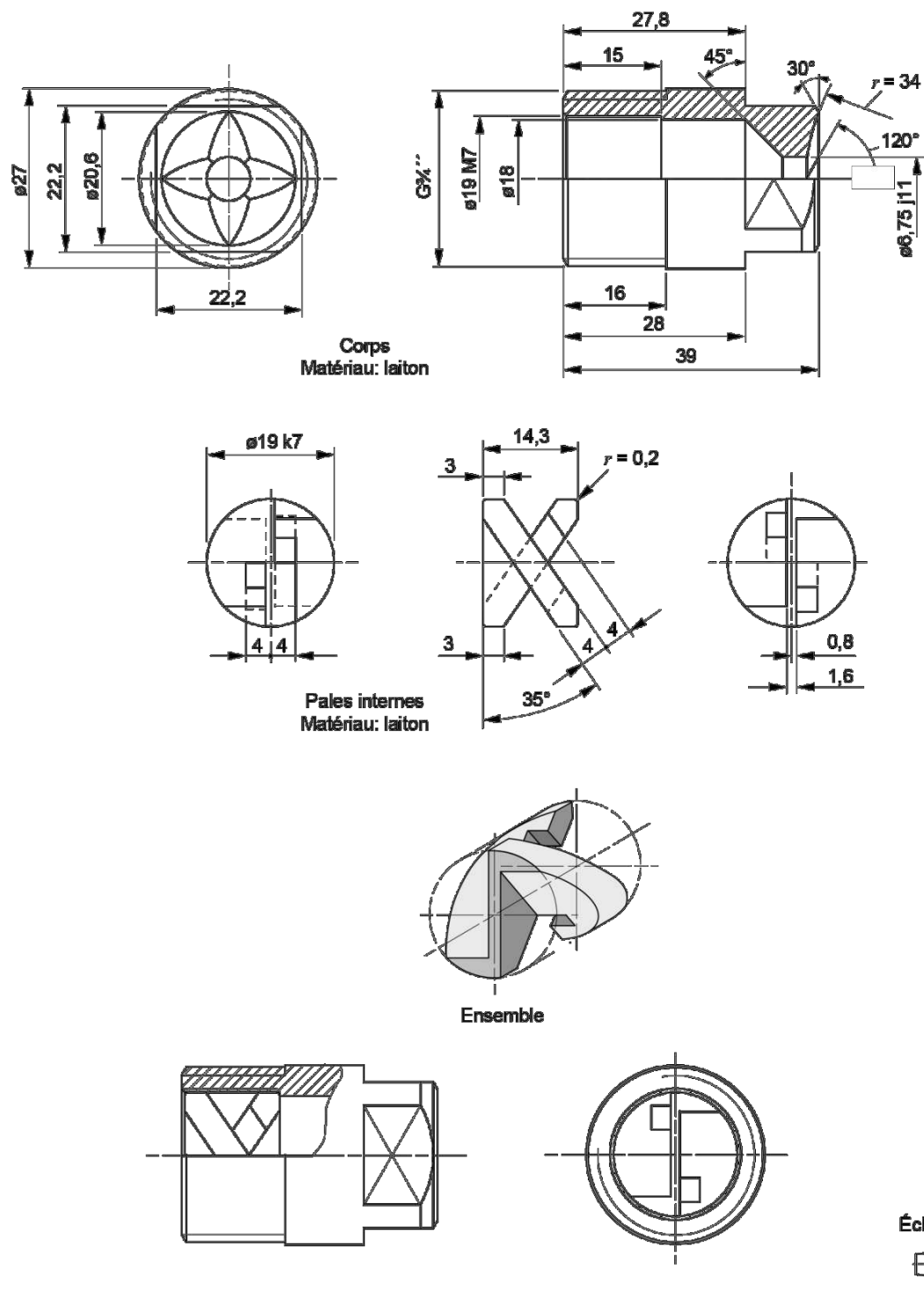
Figure C.2 – Buse pour l'essai de protection contre les intempéries
