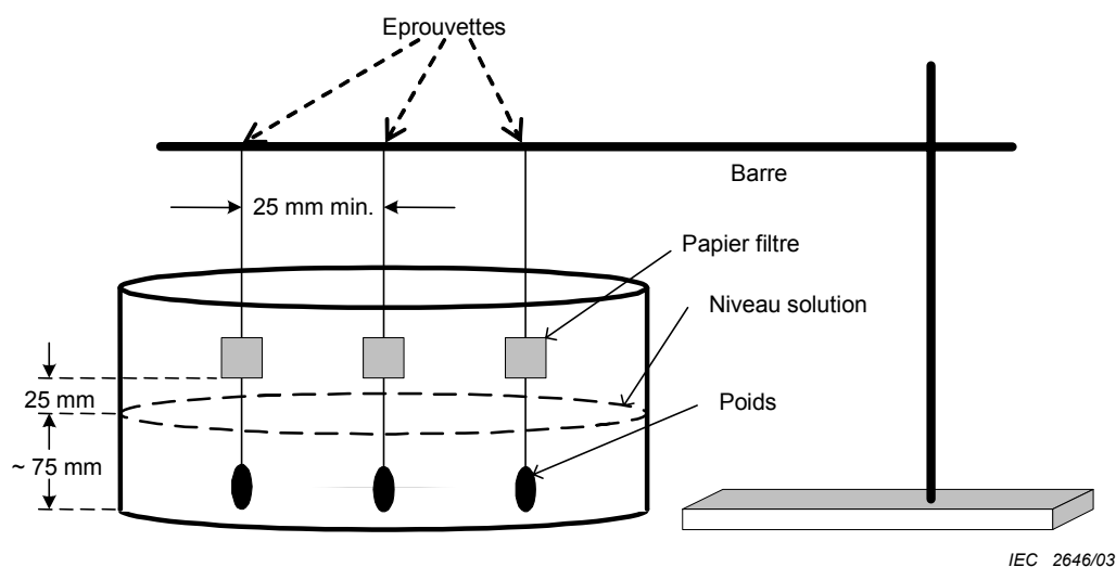
Figure 1 – Effet de mèche – Configuration de l'essai
