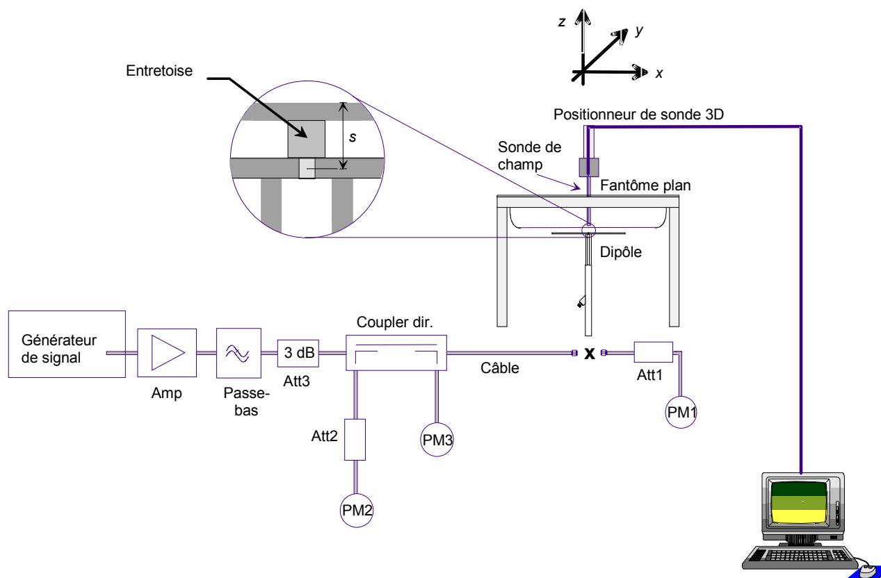
Figure B.1 – Montage pour le contrôle du système
