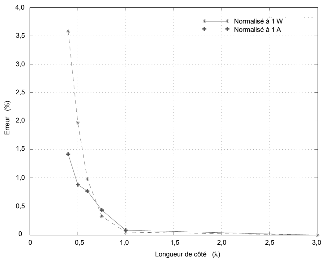
Figure D.3 – Incertitude prédite par l'utilisation d'un code FDTD pour un DAS crête spatial moyen sur 10 g, en fonction des dimensions du fantôme plan comparativement à un fantôme plan infini
