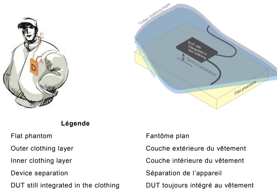
Figure 11 – Position d'essai pour les appareils sans fils intégrés aux vêtements
