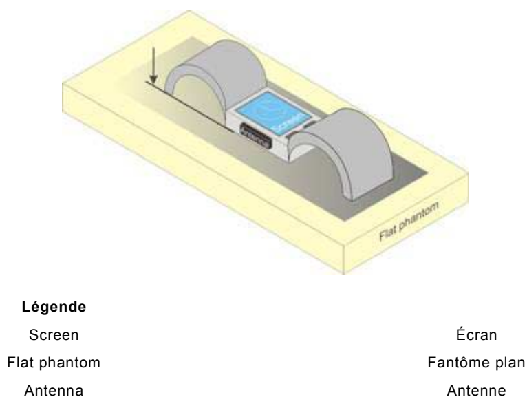
Figure 10 – Position d'essai pour les appareils fixés à un membre
