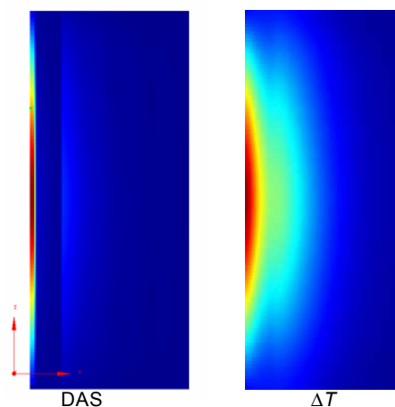
Figure H.1 – Distributions du DAS et de l'augmentation de température ( \Delta T ) simulées pour un modèle de torse plan à trois couches (peau, graisse, muscle)
