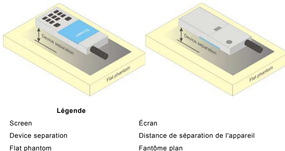
Figure 5 – Positions d'essai pour les appareils portés près du corps
