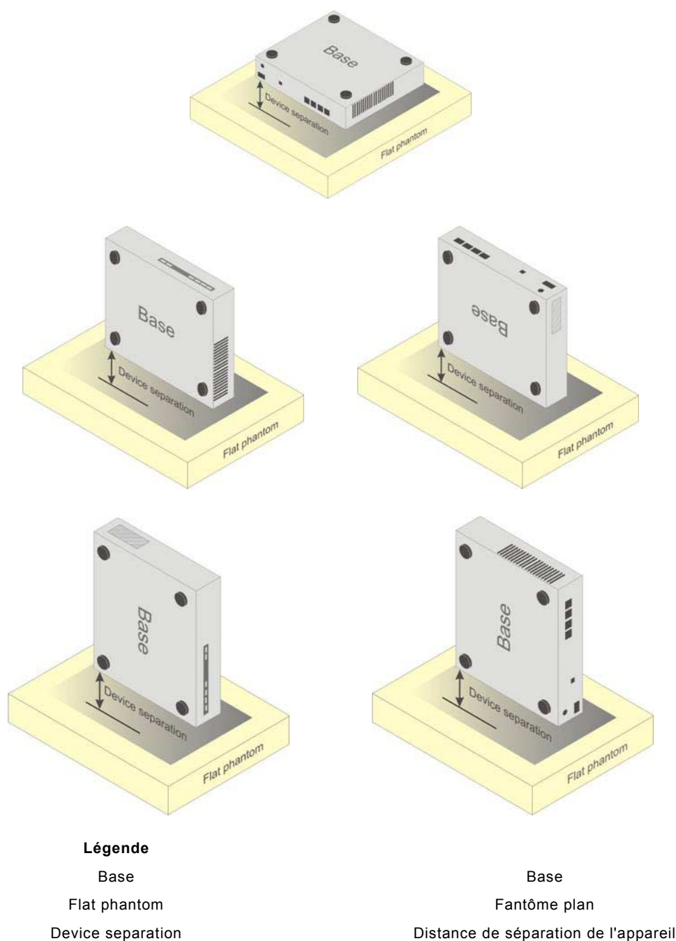
Figure 8 – Positions d'essai pour les appareils de bureau
