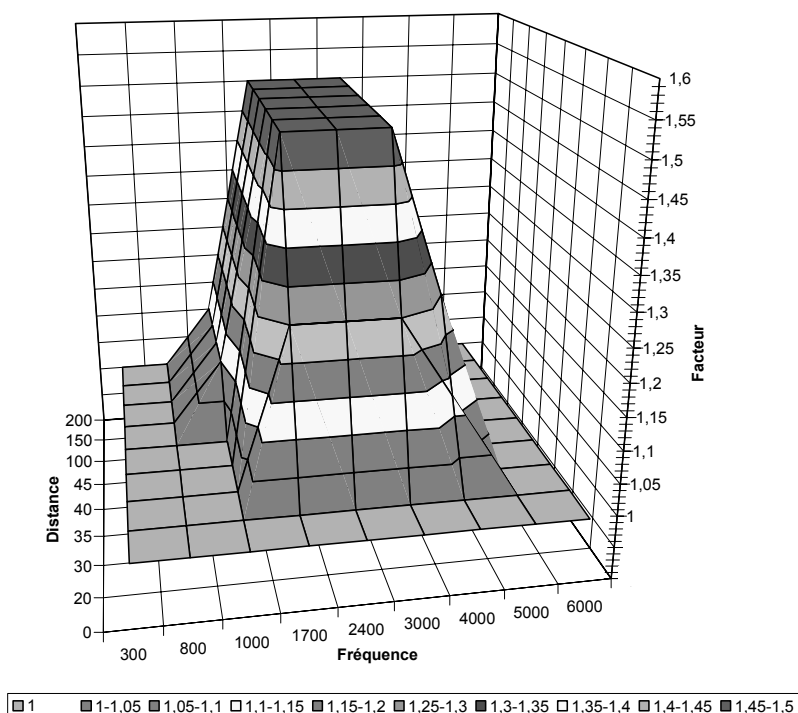
Figure H.3 – Facteurs d'amélioration pour la peau du DAS moyen
