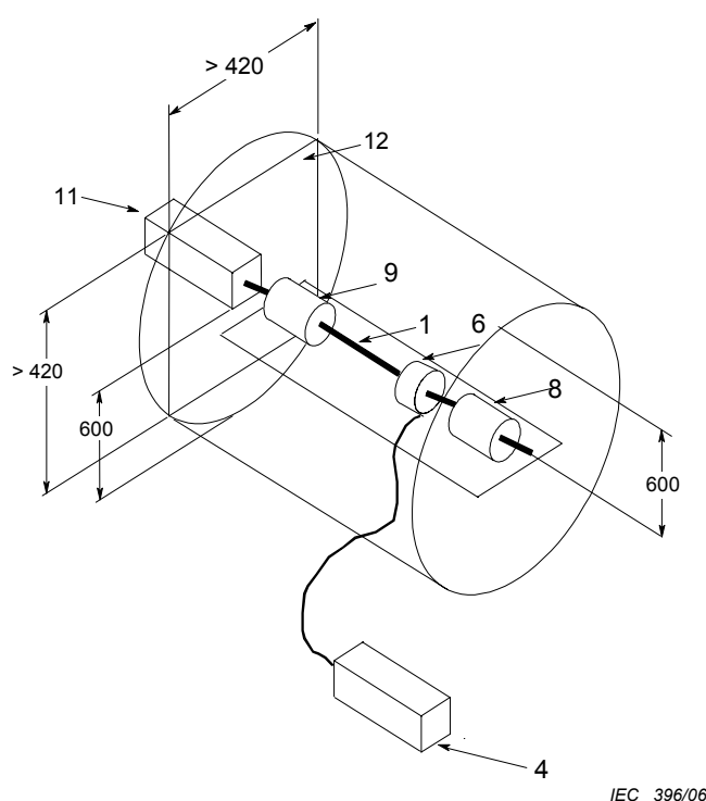
Figure 13 – Disposition de blindage pour une mesure d'extrémité la plus éloignée
