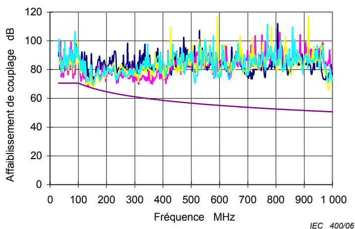
Figure 17 – Erreur de mesure fréquente d'un câble symétrique
