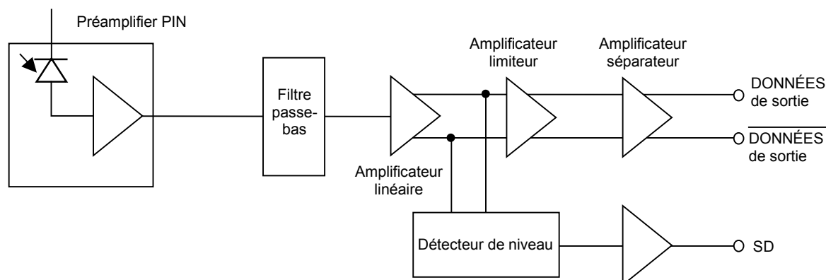
Figure 1 – Diagramme schématique de la section du récepteur
