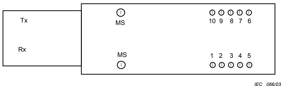
Figure 1 – Attribution des numéros des bornes électriques (vue du dessus avec les broches en dessous)
