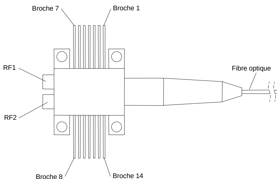
Figure 1 – Affectation du numérotage de bornes électriques pour les composants émetteurs munis de connecteurs coaxiaux RF doubles
