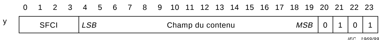
Figure 4 – Structure de la trame de synchronisation
