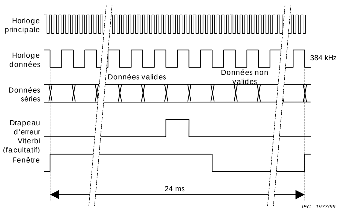
Figure A1 – Signaux logiques de l'interface DAB3
