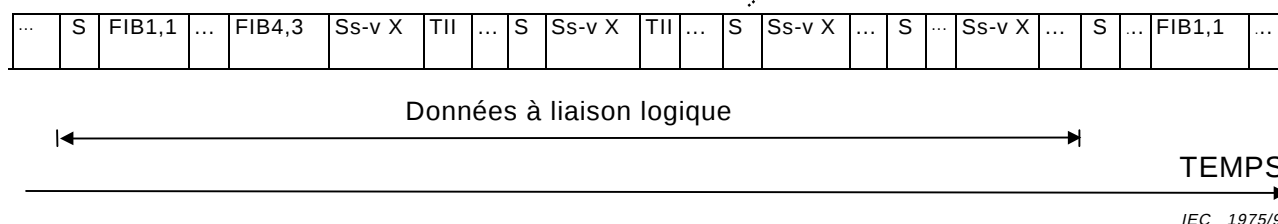
Figure 10 – Ordre de transmission sur RDI (exemples)
