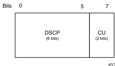
Figure C.3 – Format du paramètre de la classe Traffic
