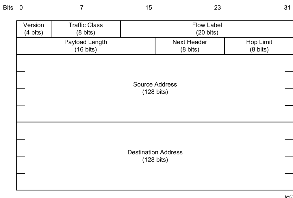
Figure C.2 – Format d'en-tête IPv6
