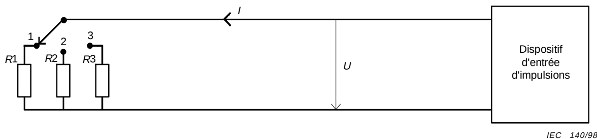
Figure D.1 – Circuit d'essai du dispositif d'entrée d'impulsions
