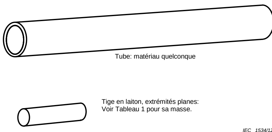
Figure 2 – Constituant du dispositif d'essai de choc
