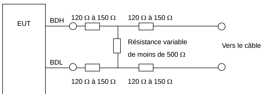
Figure 124 – Circuit d'essai de forme d'onde d'entrée minimale
