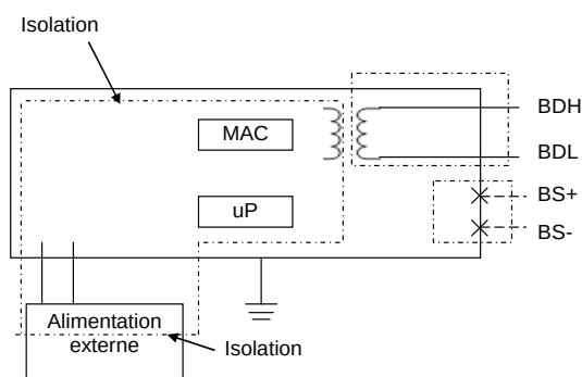
Figure 82 – Exemple d'isolation d'un esclave non alimenté par le réseau
