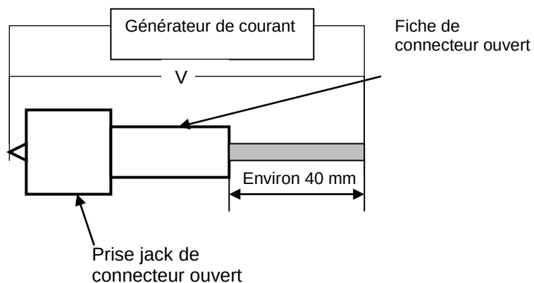
Figure 107 – Méthode de mesure de la résistance de contact (connecteurs ouverts)
