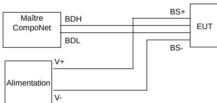
Figure 120 – Connexion inversée de la ligne d'alimentation
