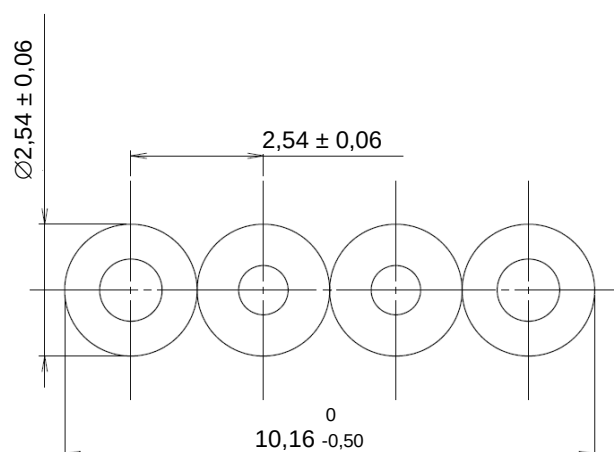
Figure 98 – Dimension du câble plat I
