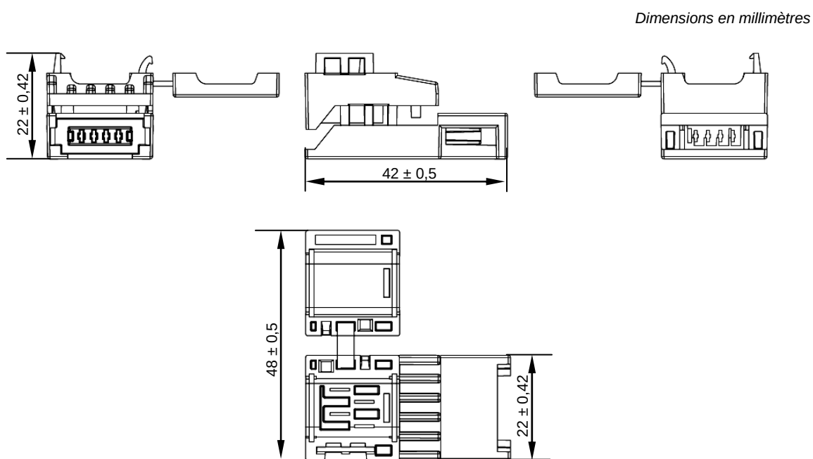
Figure 112 – Fiche de connecteur plat II (informative)
