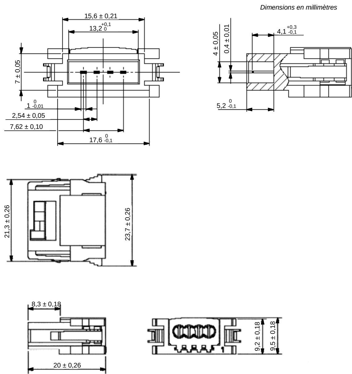
Figure 109 – Fiche de connecteur plat I
