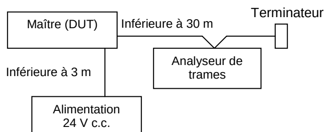
Figure 127 – Configuration d'essai de trafic minimal d'un DUT maître
