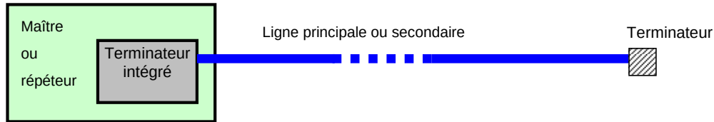
Figure 84 – Position d'un terminateur
