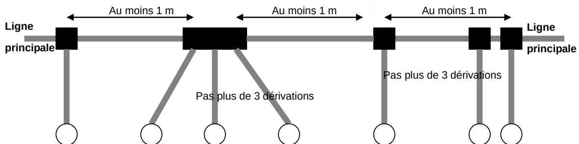
Figure 87 – Restriction pour les dérives
