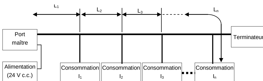
Figure 117 – Chute de tension sur un câble donné
