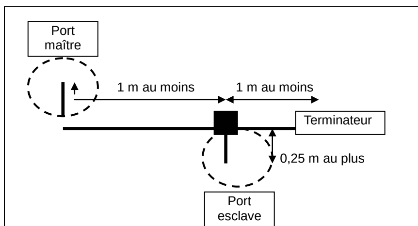
Figure 125 – Système d'essai de forme d'onde d'entrée minimale
