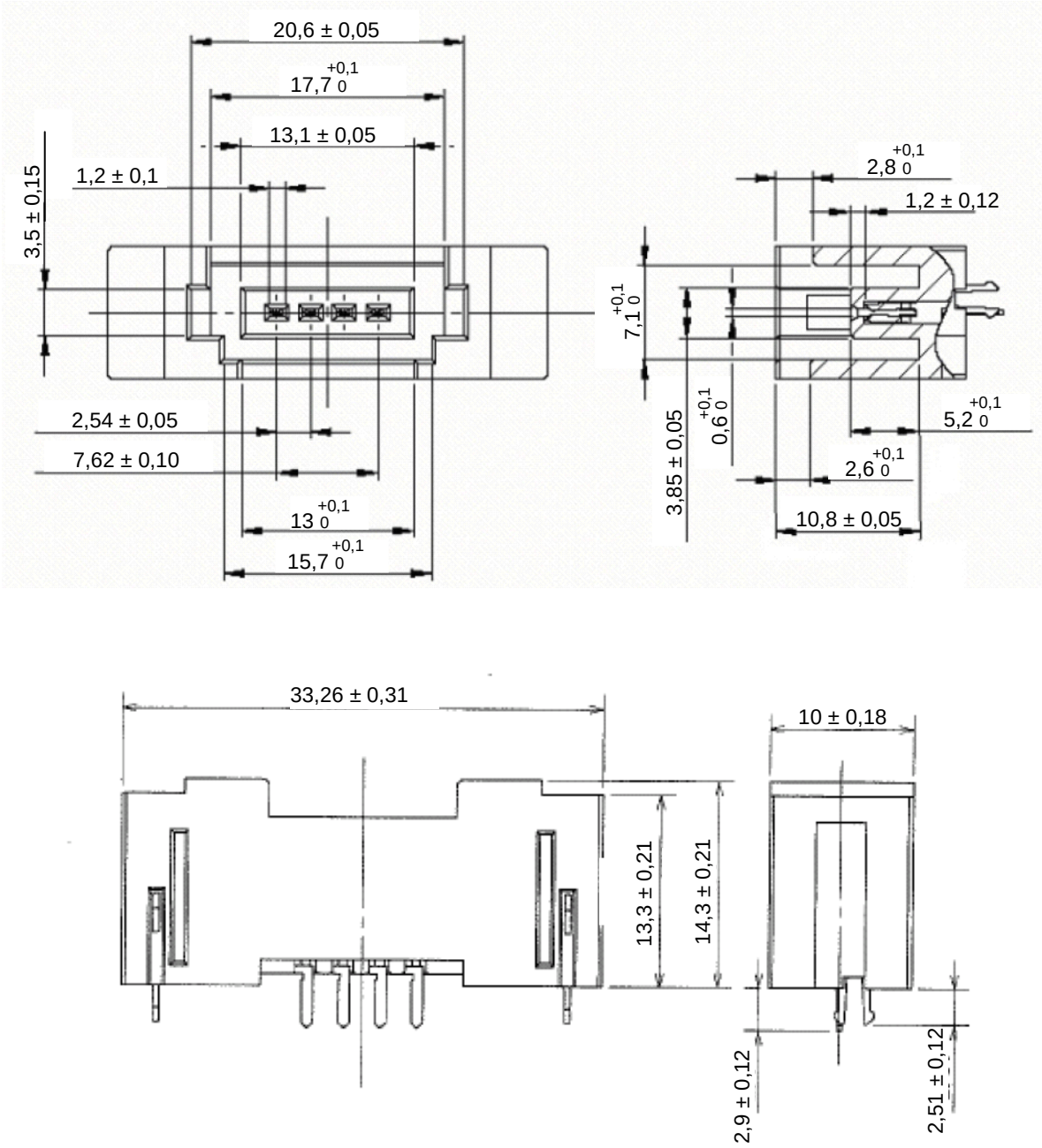
Figure 106 – Prise jack de connecteur ouvert (informative)
