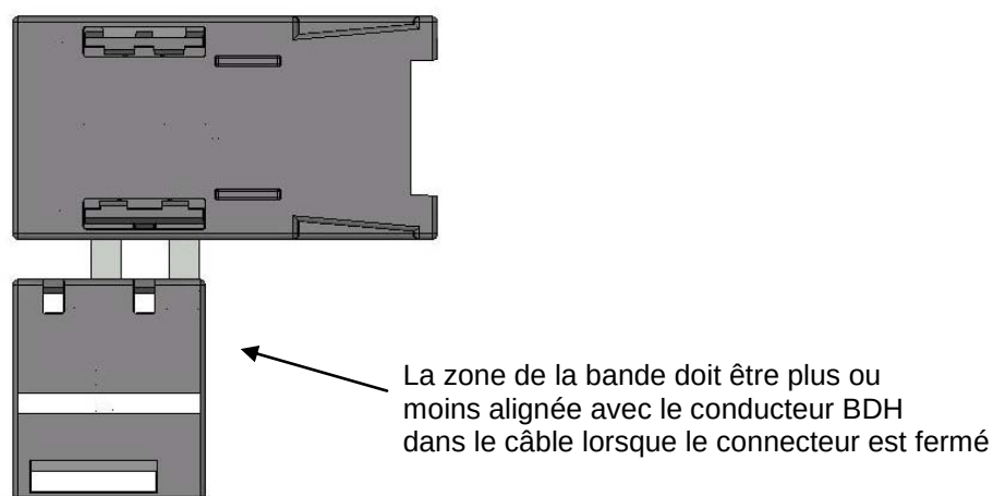
Figure 114 – Marquage de connecteur pour lignes principales
