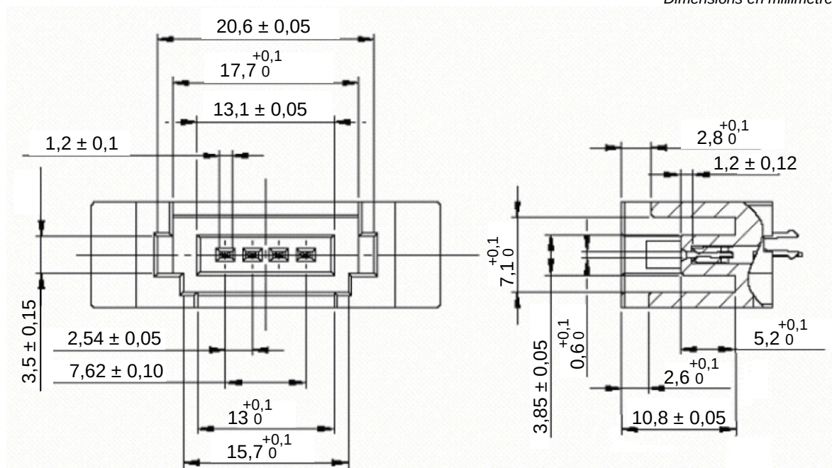
Figure 103 – Dimensions d'accouplement des connecteurs à prise jack
