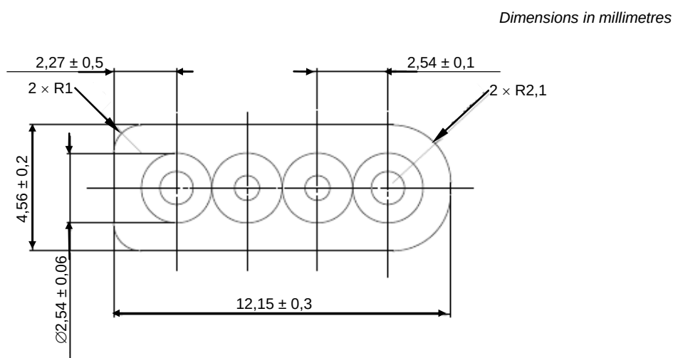
Figure 100 – Dimension du câble plat II
