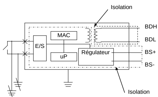
Figure 81 – Exemple d'isolation d'un simple esclave nécessitant une connexion à des appareils ayant un câblage de signalisation non mis à la masse
