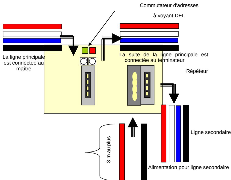
Figure 94 – Segments de réseau alimentés par des répéteurs
