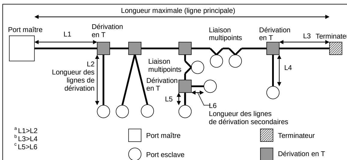
Figure 89 – Méthode de câblage d'usage général
