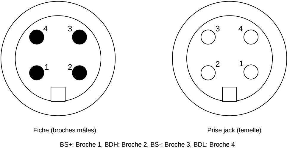
Figure 115 – Configuration de broches de connecteur M12
