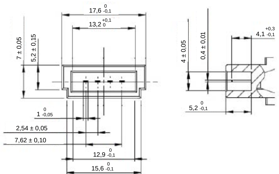
Figure 101 – Dimensions d'accouplement du connecteur à fiche
