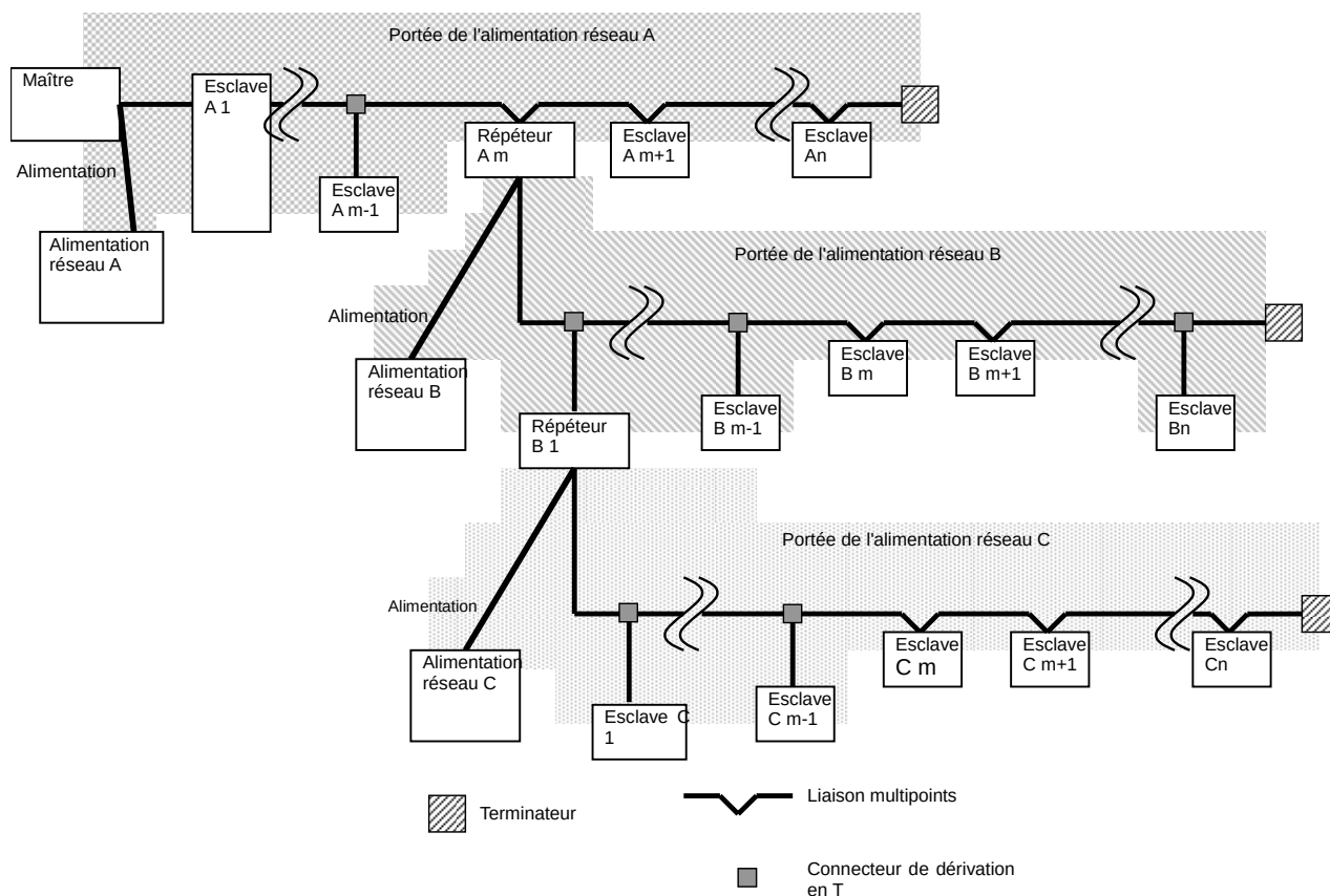
Figure 91 – Méthode de distribution de l'alimentation
