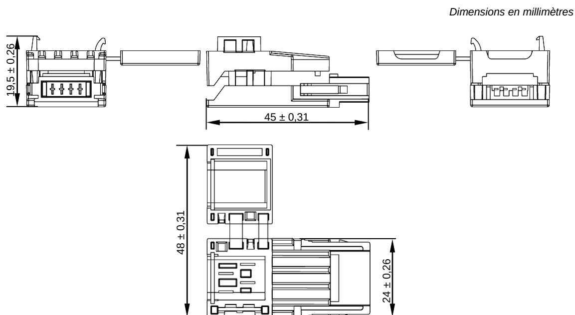
Figure 112 – Fiche de connecteur plat II (informative)
