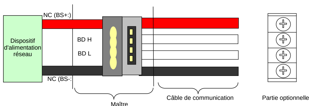
Figure 93 – Connexion à la source d'alimentation
