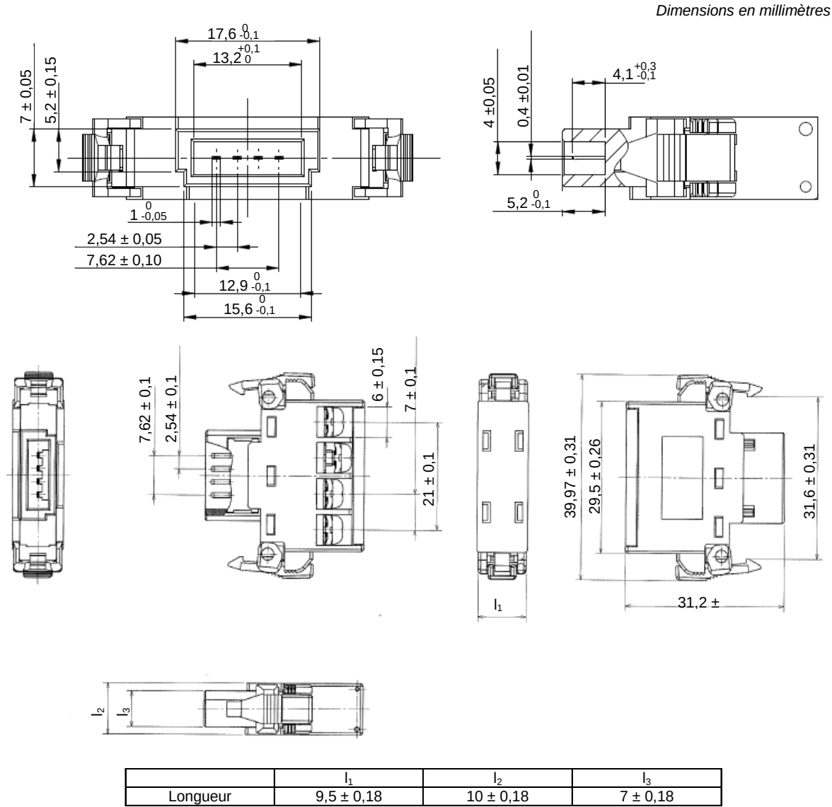
Figure 105 – Fiche de connecteur ouvert (informative)
