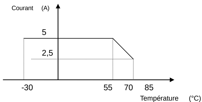
Figure 108 – Courant de déclassement des connecteurs
