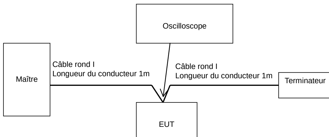
Figure 123 – Circuit d'essai du port esclave d'un esclave de données de sortie
