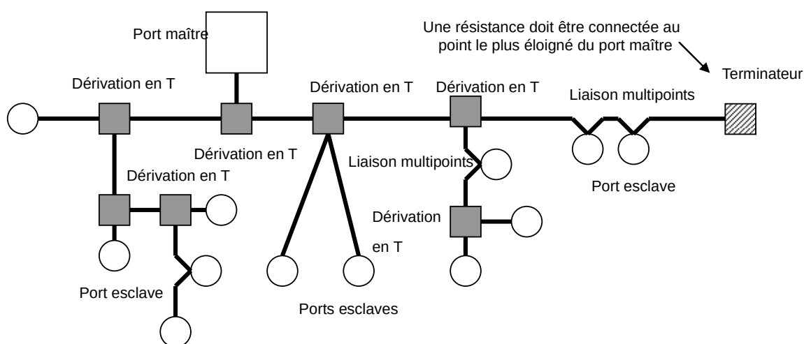
Figure 90 – Méthode de câblage souple
