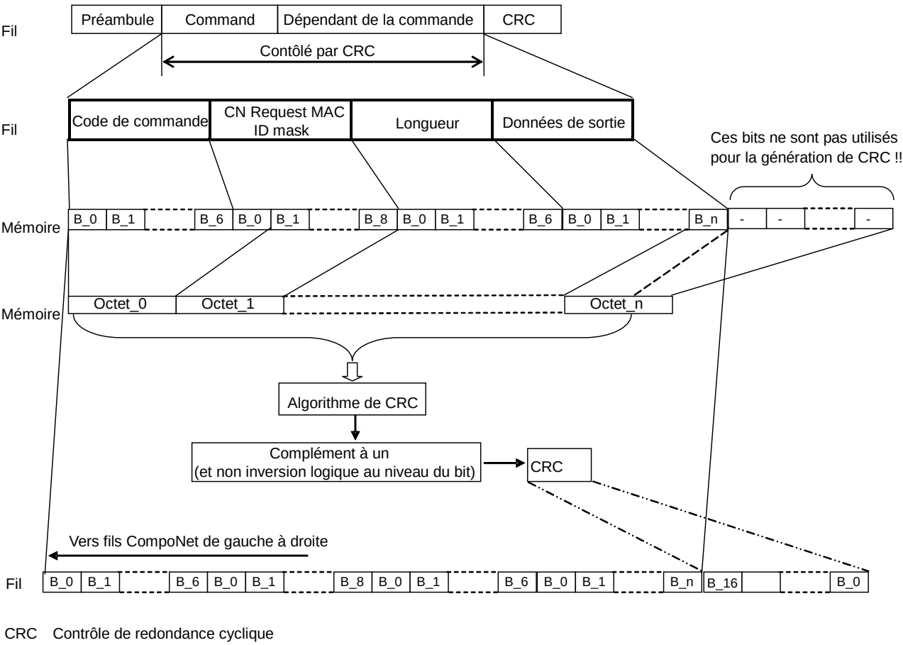
Figure D.1 – Exemple de génération de CRC
