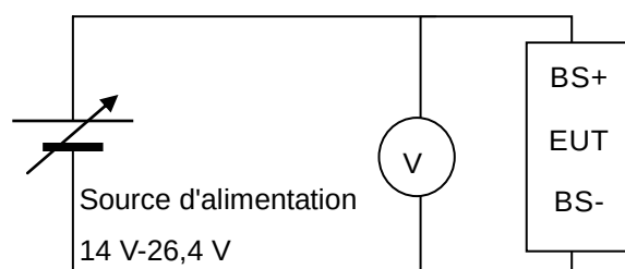
Figure 119 – Circuit d'essai de la tension de fonctionnement
