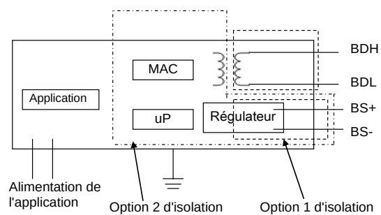
Figure 80 – Exemple d'isolation d'un module E/S avec connectivité à d'autres sources d'alimentation
