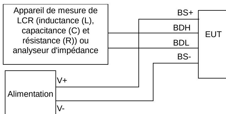
Figure 122 – Impédance d'entrée
