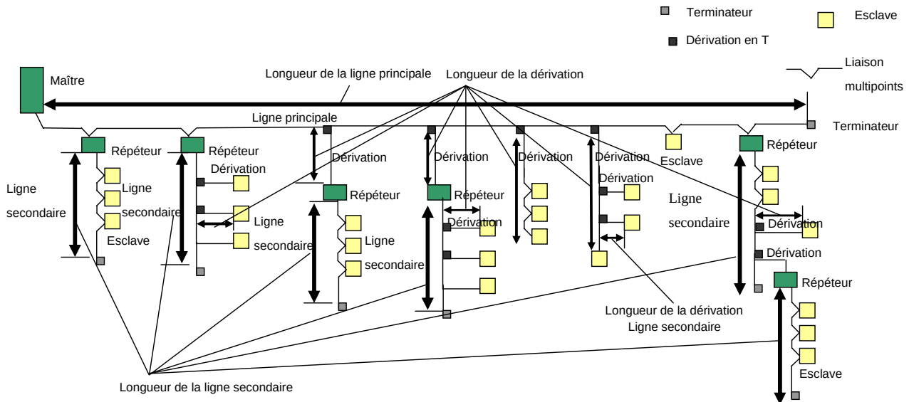
Figure 86 – Illustration des restrictions en matière de longueur du câblage
