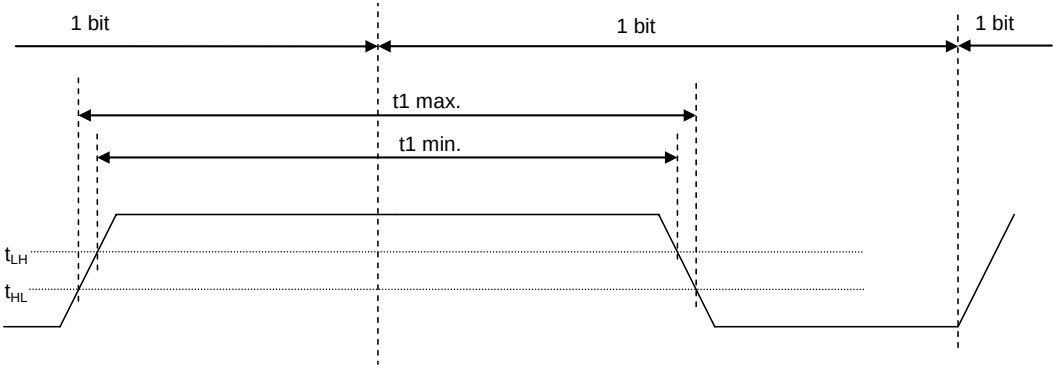
Figure 71 – Masque de réception numérique 2
