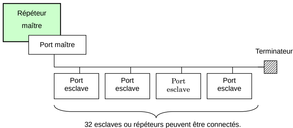
Figure 85 – Nombre d'appareils par segment
