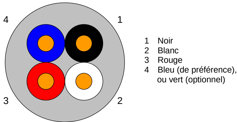
Figure 96 – Aperçu du câble rond II
