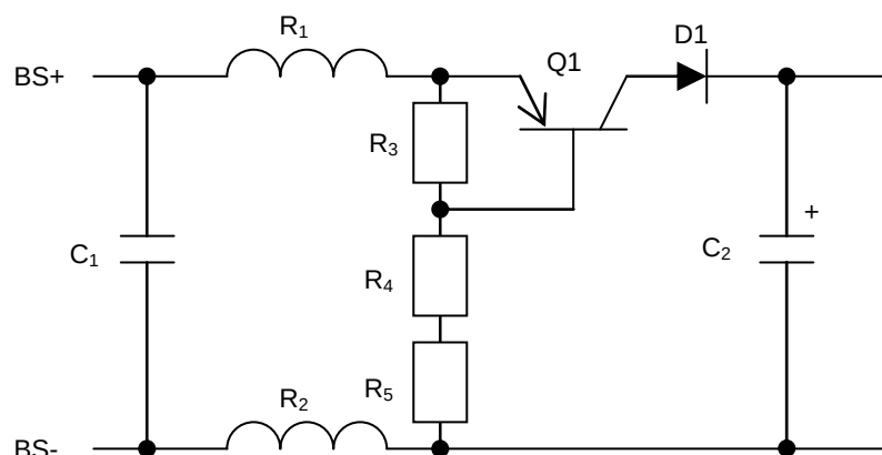
Figure 118 – Conception de l'alimentation d'une station (informative)
