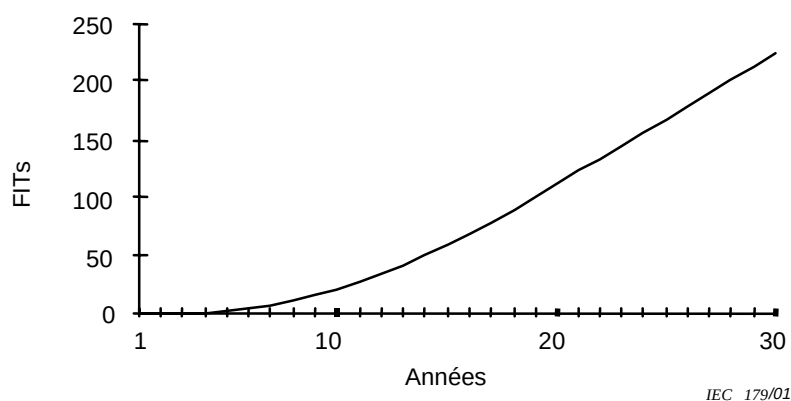
Figure 6 – Fiabilité de composant en service
