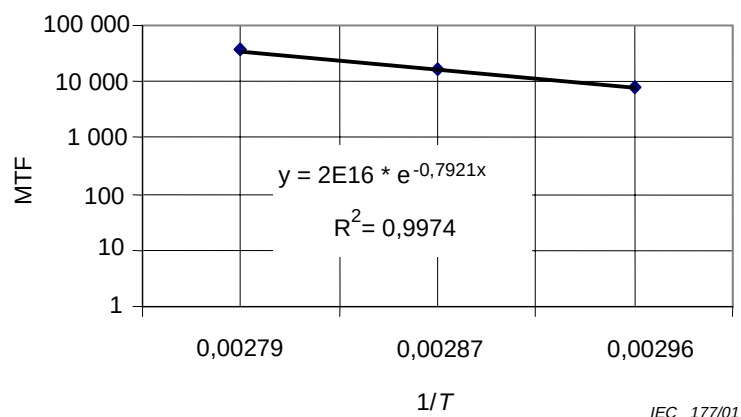
Figure 4 – Ajustement de la courbe exponentielle pour MTF par rapport à 1/T
