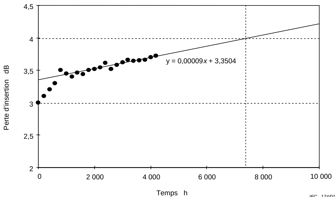
Figure 1 – Extrapolation des résultats pour la détermination de la durée de fonctionnement avant défaillance
