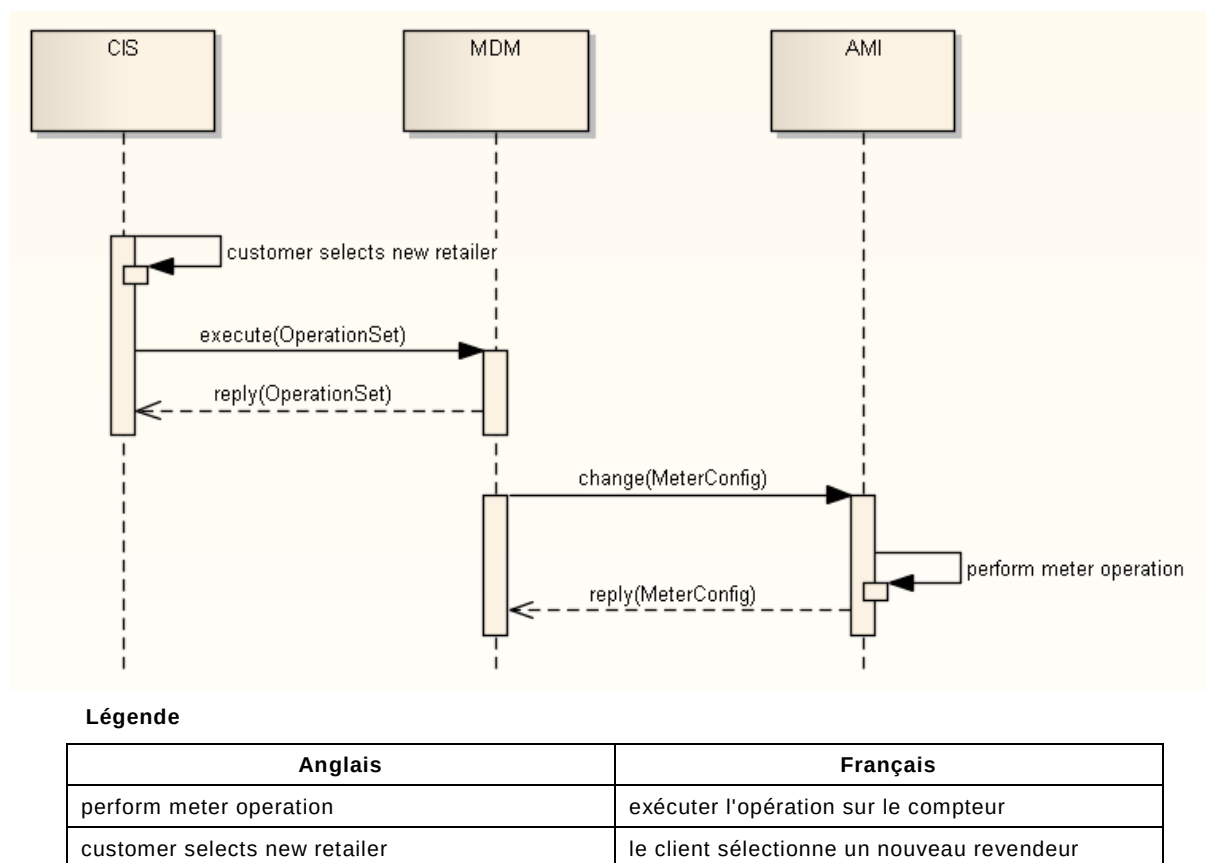
Figure 43 – Exemple d'échange de message de commutation clientèle
