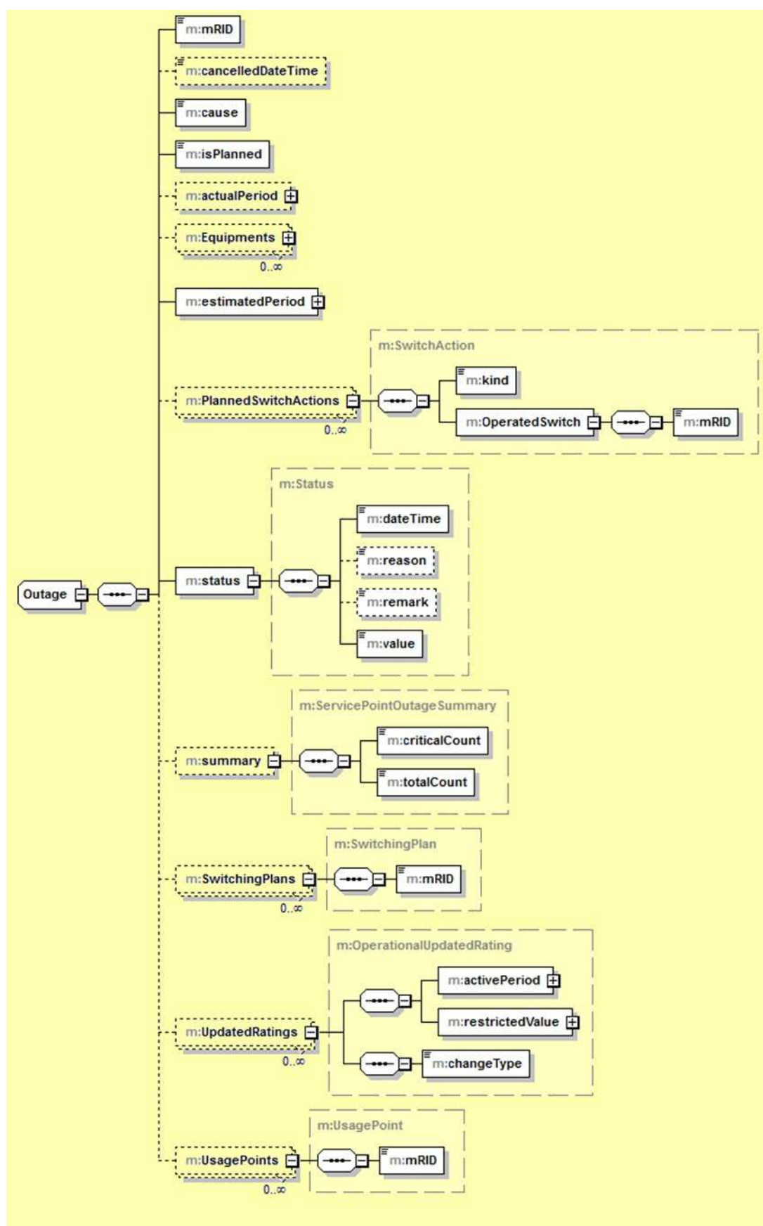
Figure 42 – Charge utile de message OutageSchedule, détails de PlannedOutages
