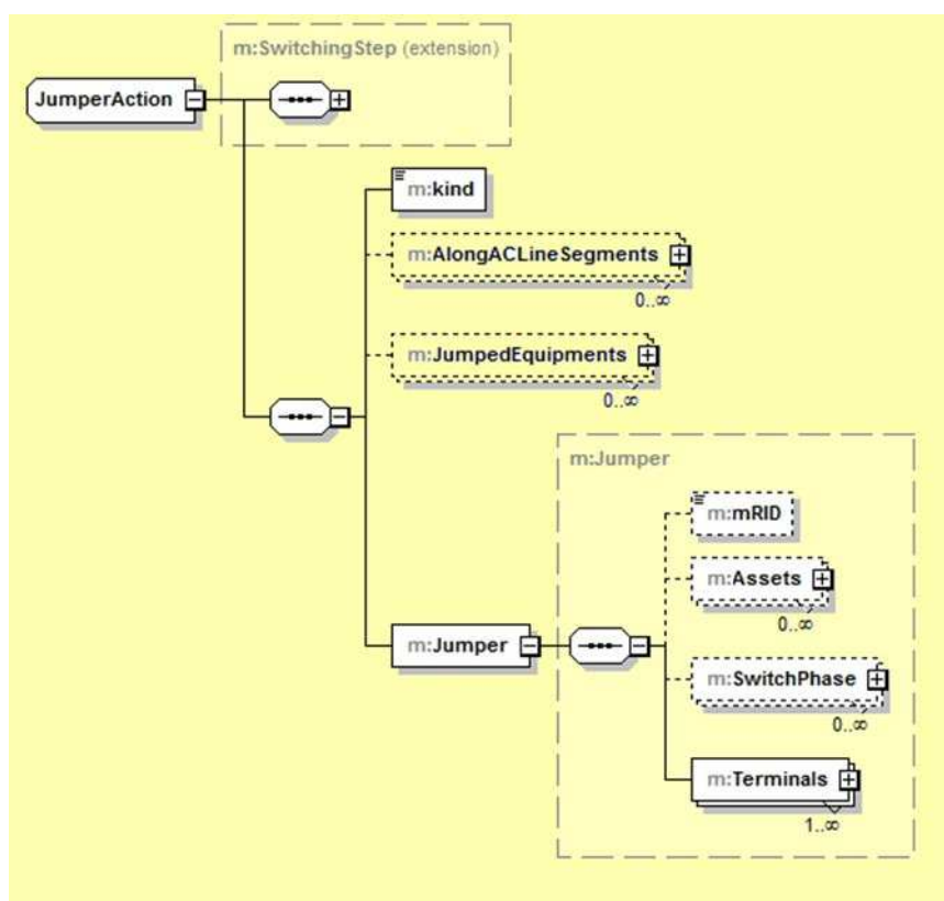
Figure 23 – Charge utile de message SwitchingPlan , détails de JumperAction
