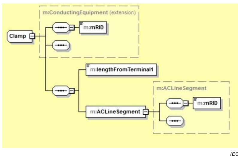
Figure 10 – Charge utile de message TemporaryNetworkChanges, détails de Clamp
