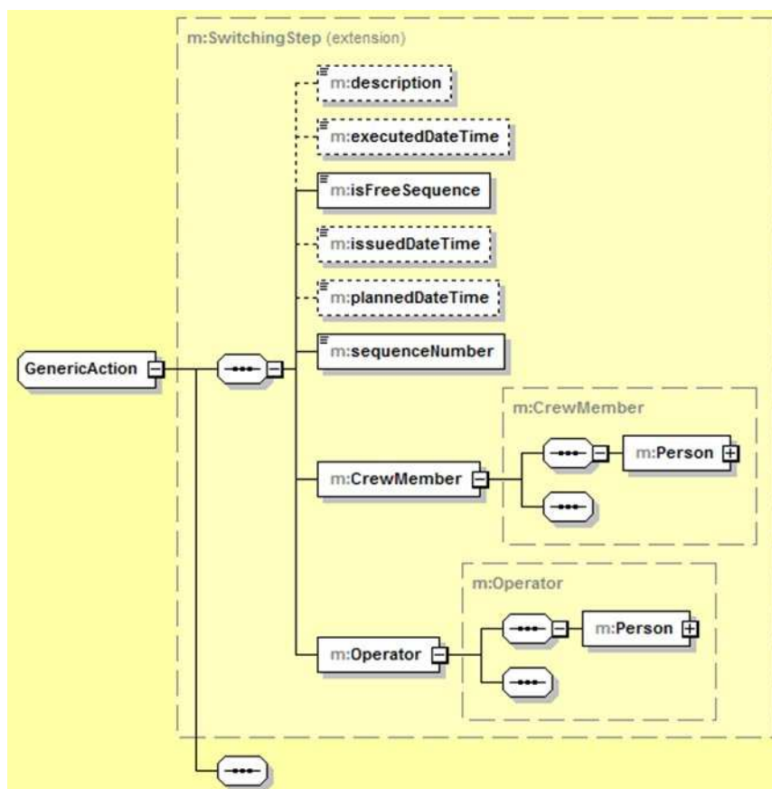
Figure 19 – Charge utile de message SwitchingPlan , détails de GenericAction
