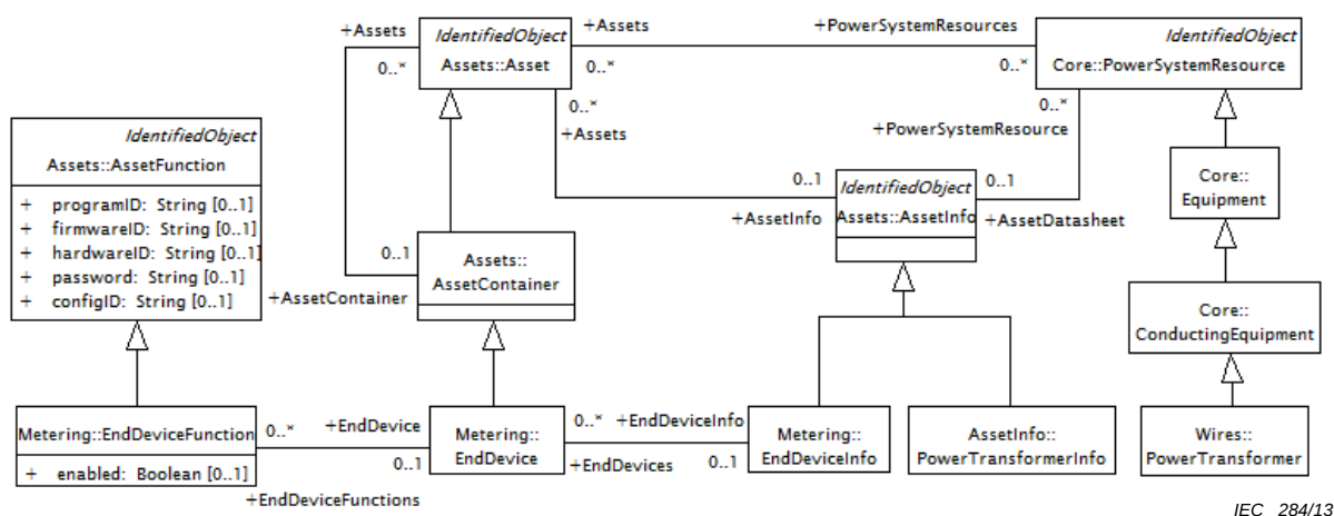
Figure 7 – Biens DCIM – lignes directrices de spécialisation
