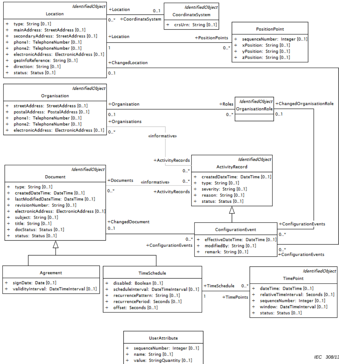
Figure 31 – Diagramme de classe Common::CommonOverview
