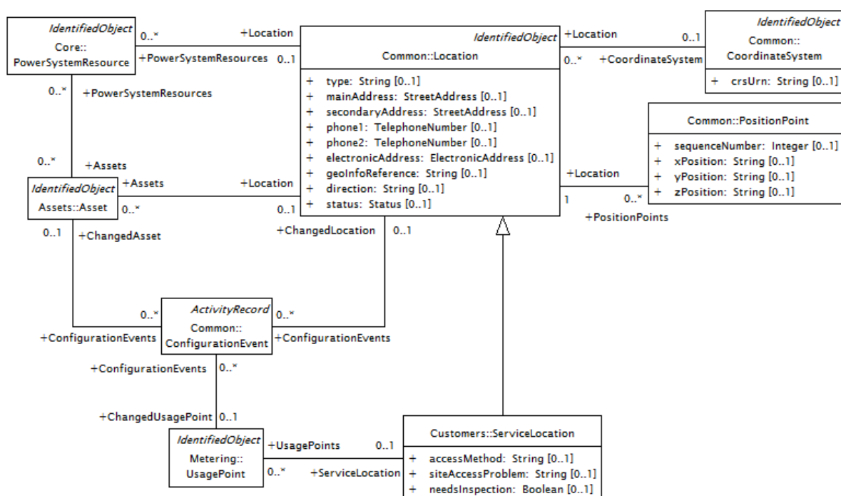
Figure 4 – Emplacements des biens et des ressources du système électrique du modèle DCIM
