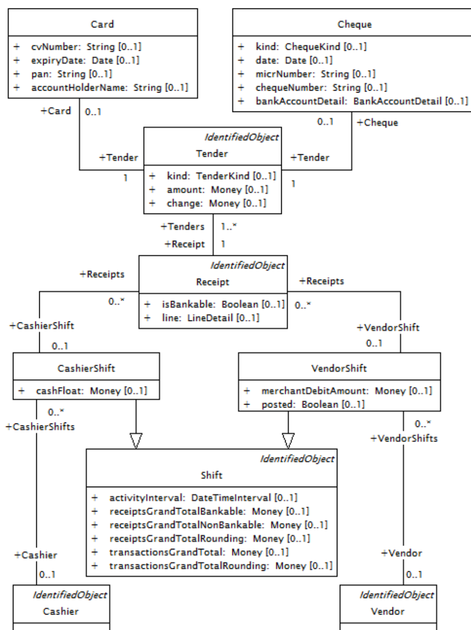
Figure 26 – Modèle d'acquittement du DCIM
