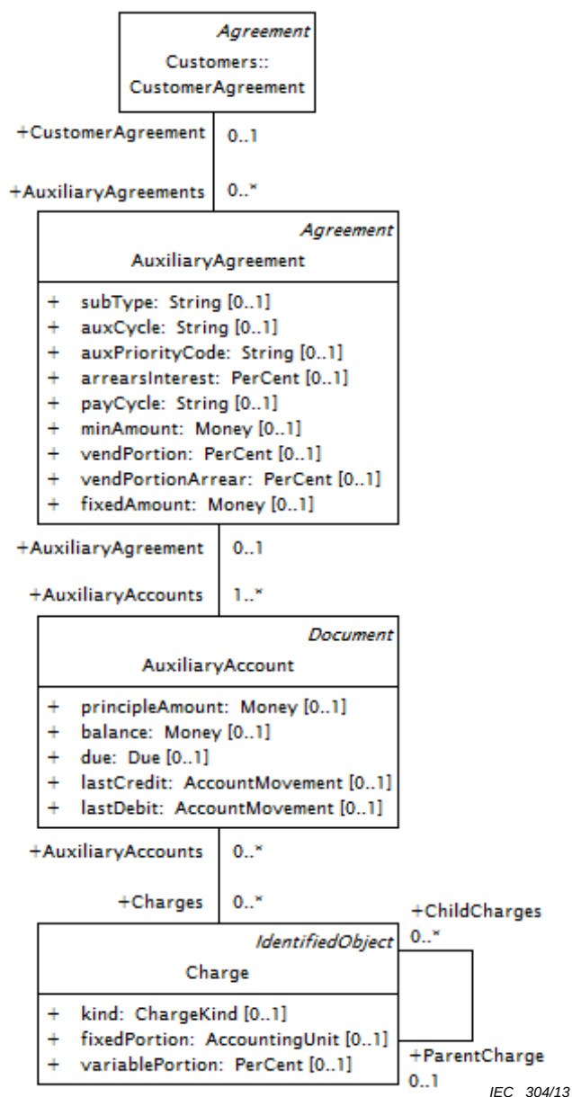
Figure 27 – Modèle d'accord auxiliaire du DCIM
