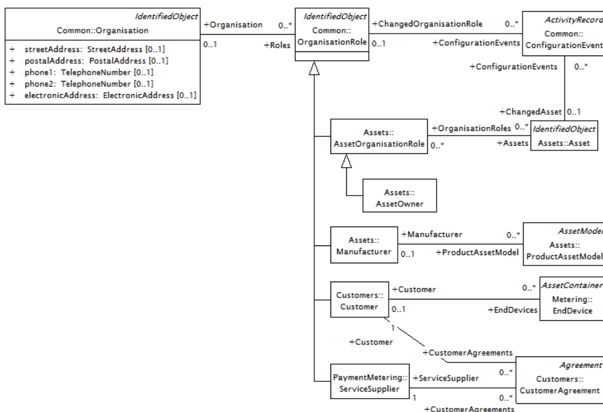
Figure 5 – Modèle d'organisation DCIM
