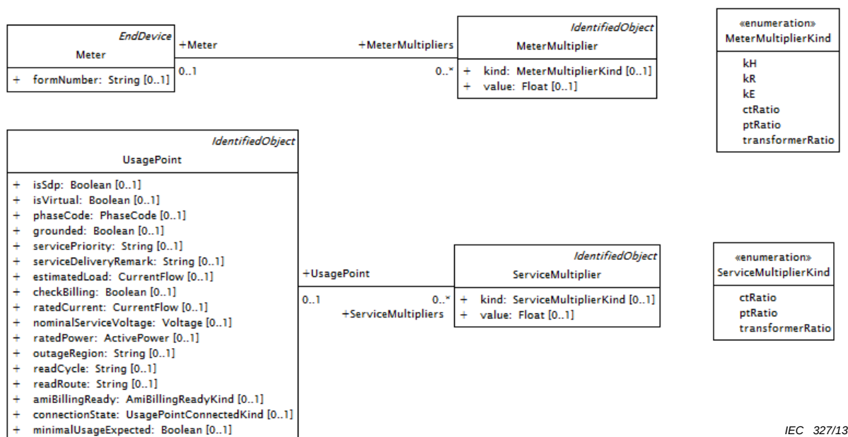
Figure 50 – Diagramme de classe Metering::MeteringMultipliers
