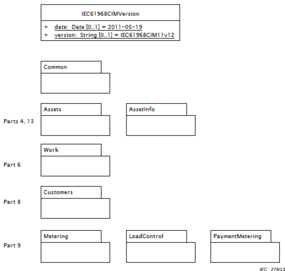
Figure 2 – Paquetages de niveau supérieur d'extensions CIM pour la distribution (DCIM)
