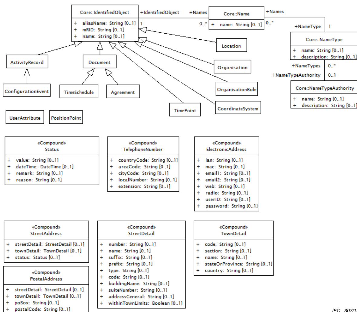
Figure 30 – Diagramme de classe Common::CommonInheritance
