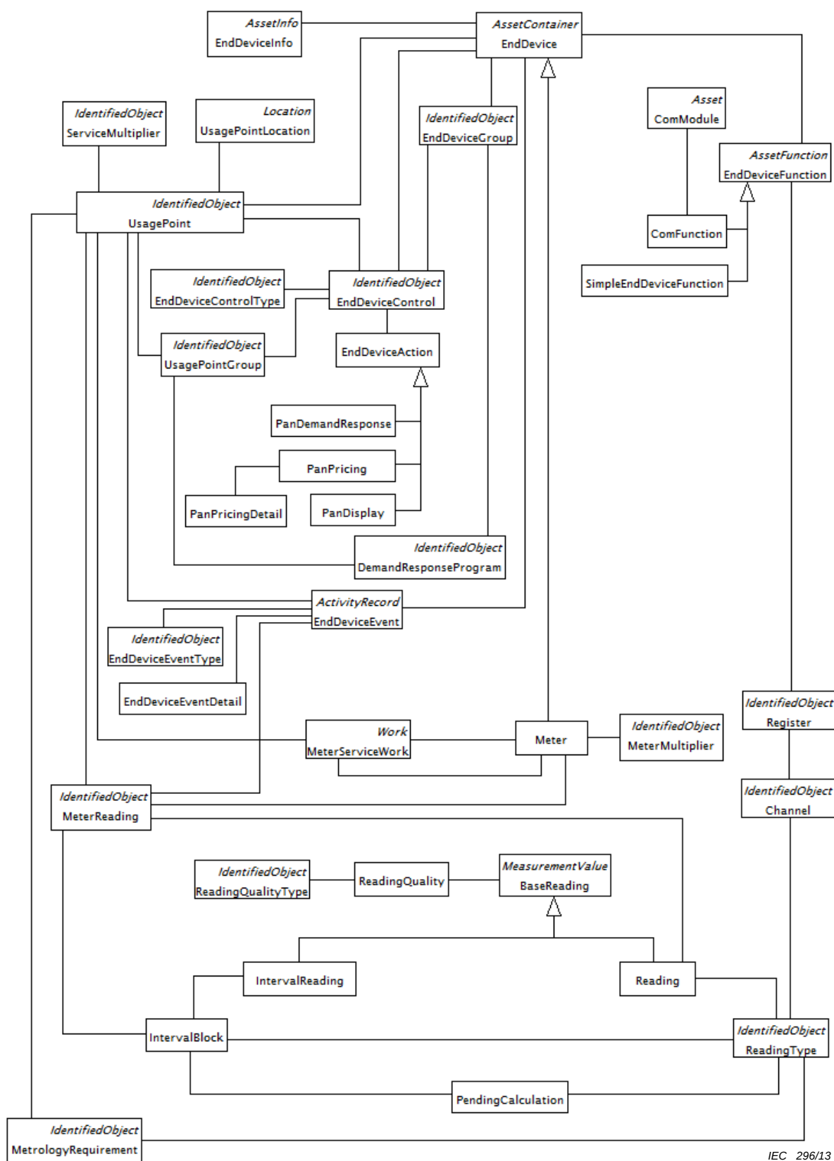
Figure 19 – Modèle de comptage du DCIM
