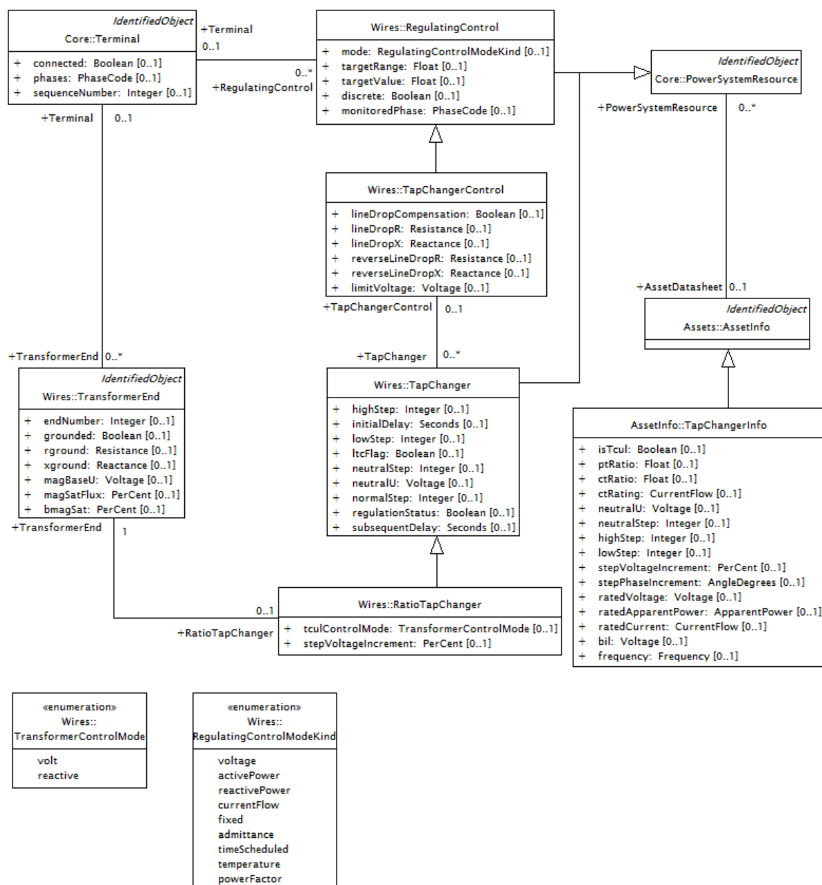
Figure 14 – Modèle de changeur de prise DCIM
