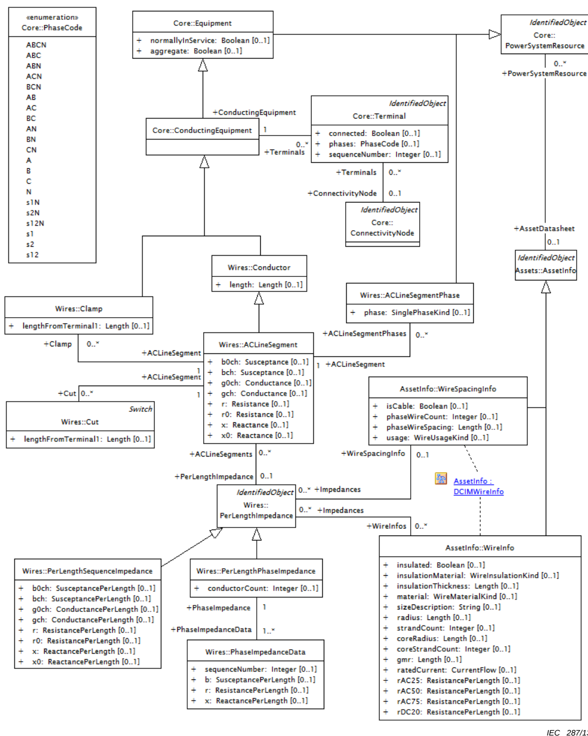
Figure 10 – Modèle de connectivité de lignes DCIM
