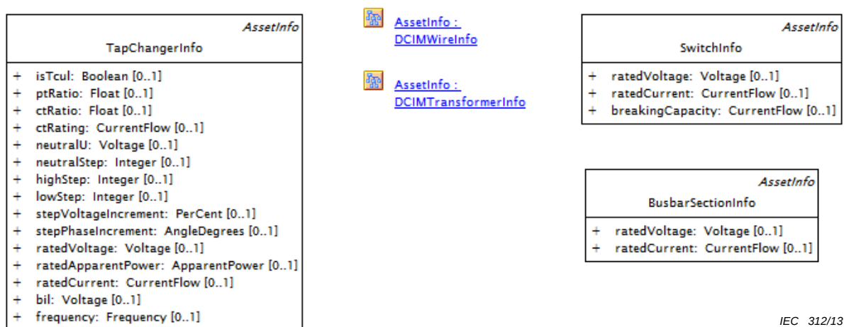
Figure 35 – Diagramme de classe AssetInfo::AssetInfoOverview
