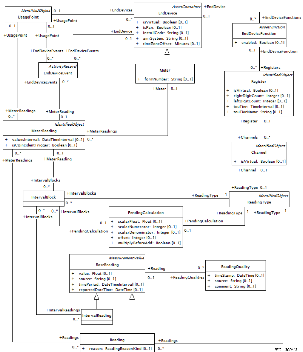
Figure 23 – Modèle de relevés de compteur DCIM
