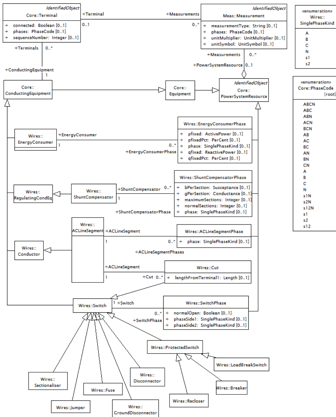
Figure 8 – Modélisation de phase DCIM
