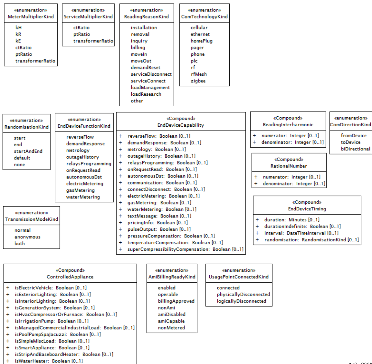
Figure 43 – Diagramme de classe Metering::MeteringDatatypes
