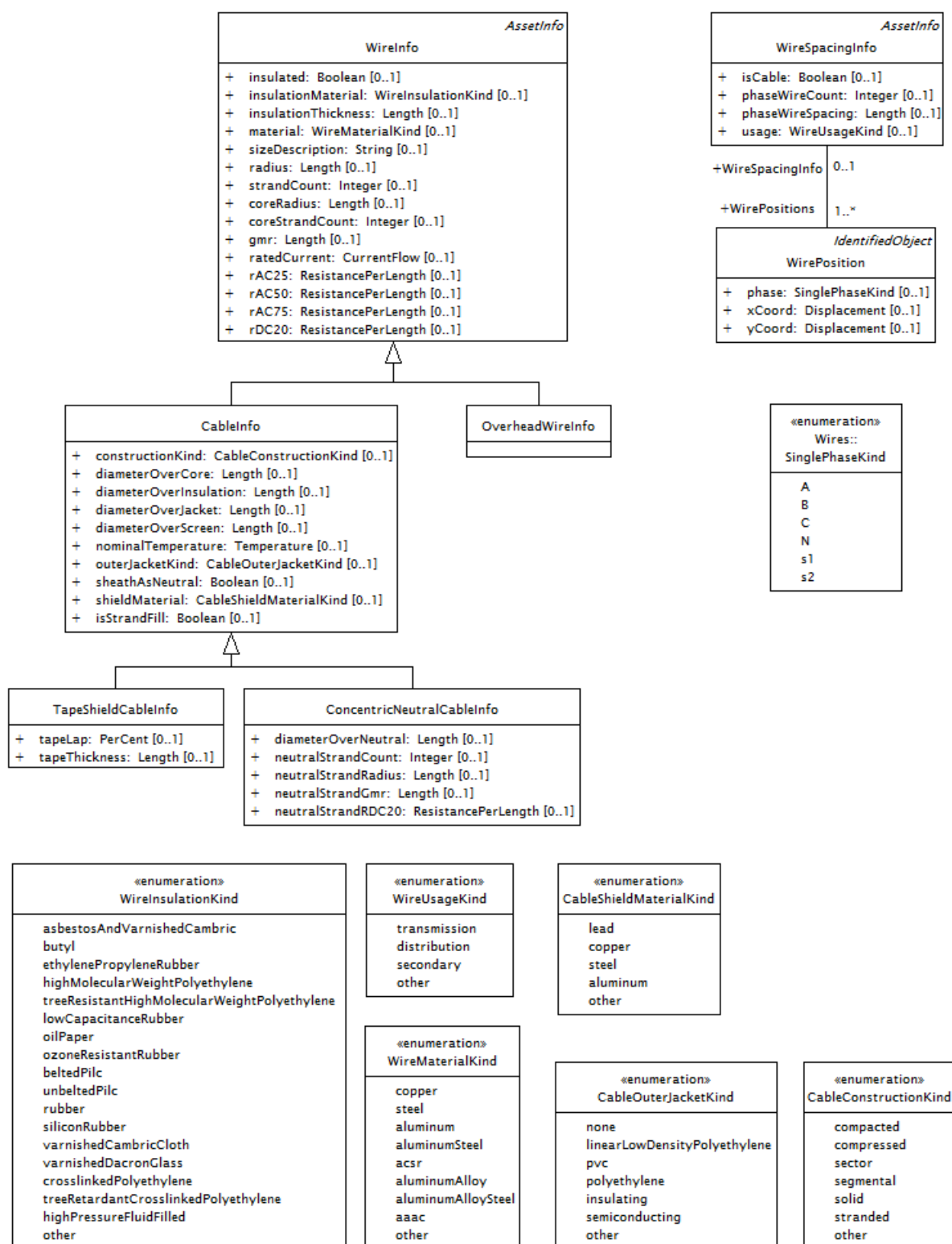
Figure 11 – Modèle (feuille de données sur les lignes et les câbles) de conducteurs DCIM
