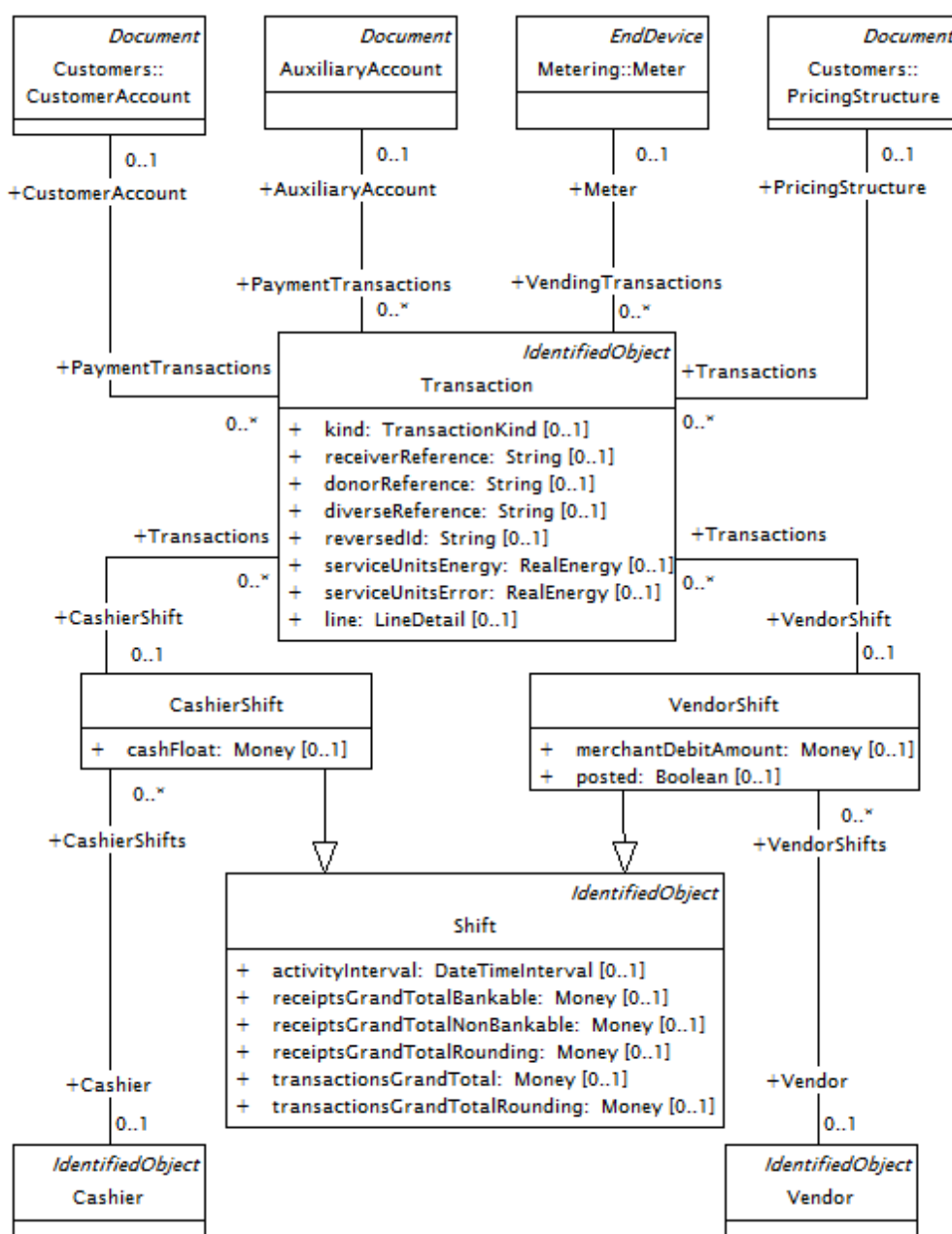
Figure 25 – Modèle de transaction du DCIM
