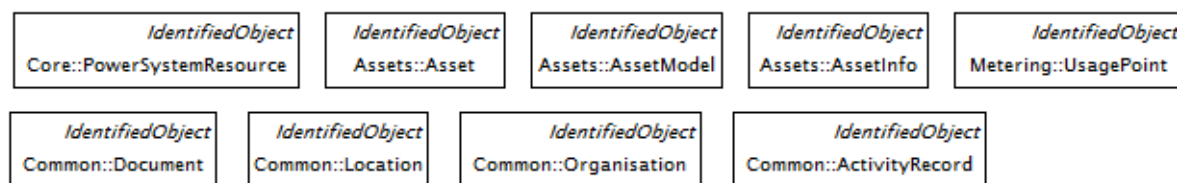
Figure 3 – Classes-clés du DCIM
