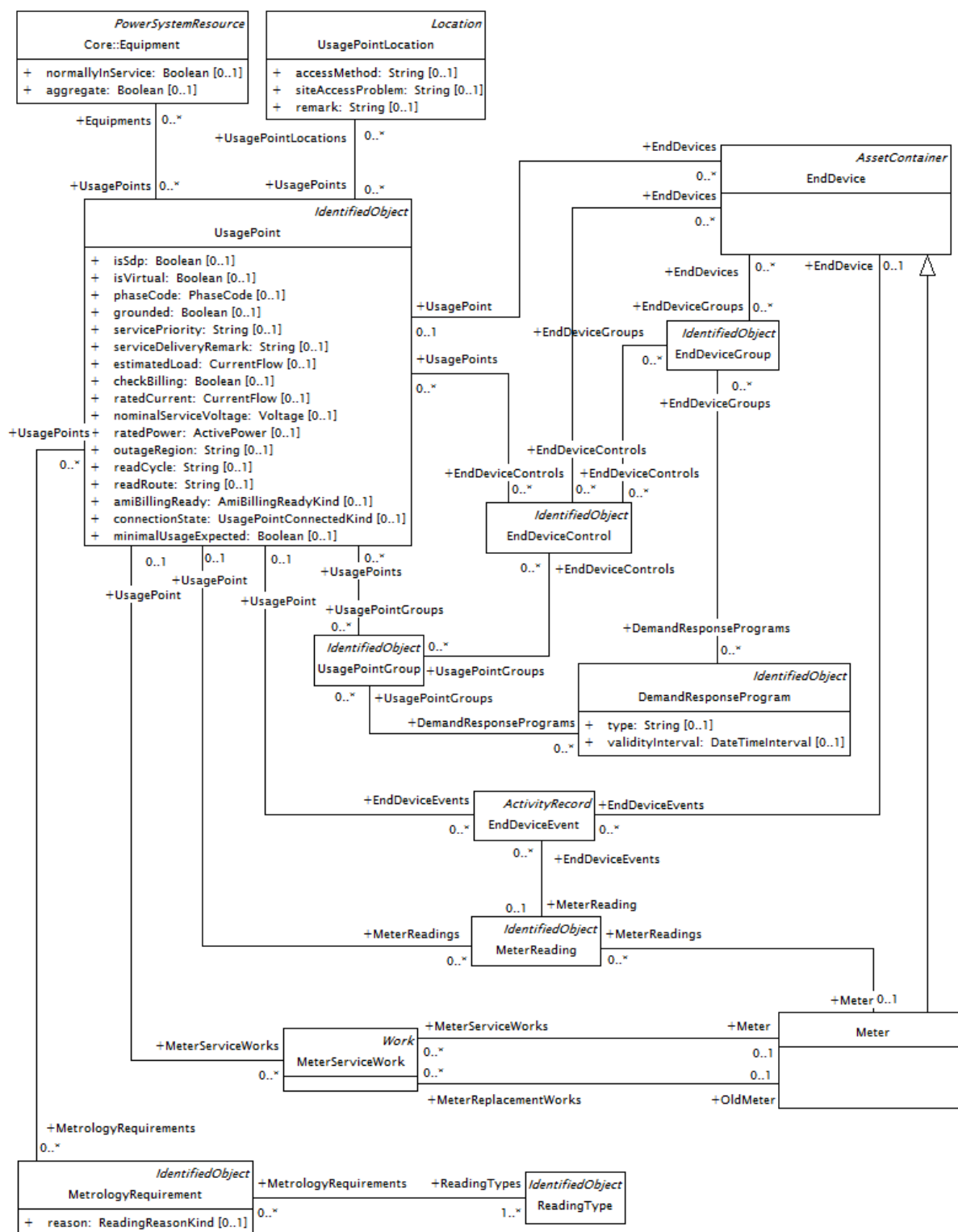
Figure 20 – Modèle de point d'usage DCIM
