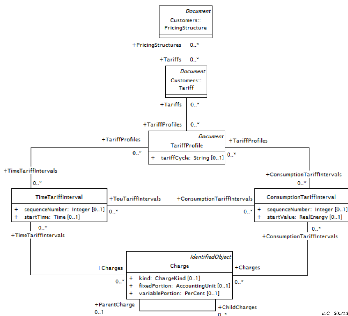
Figure 28 – Modèle de structure de tarification du DCIM
