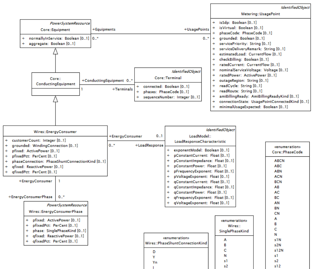
Figure 9 – Modèle de charge du DCIM
