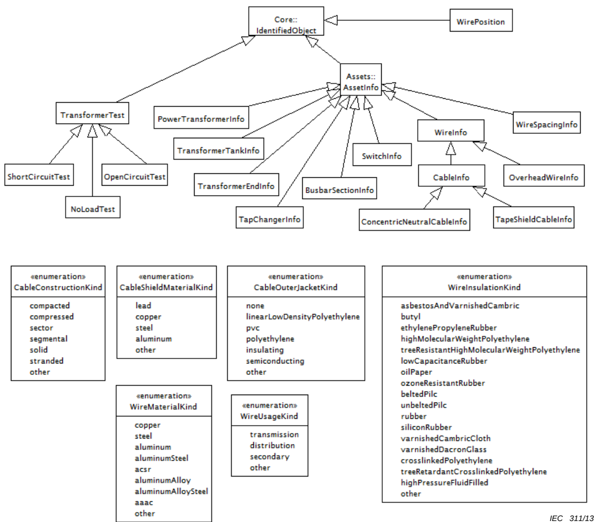
Figure 34 – Diagramme de classe AssetInfo::AssetInfoInheritance
