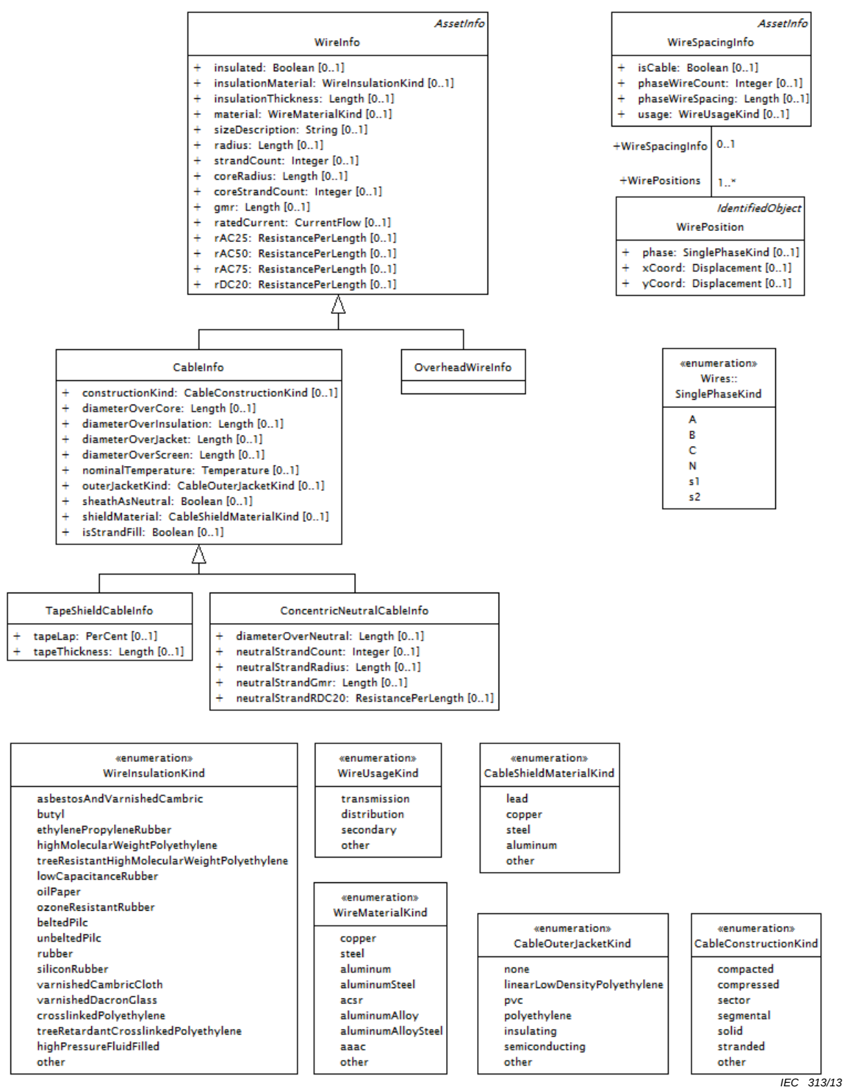
Figure 36 – Diagramme de classe AssetInfo::DCIMWireInfo
