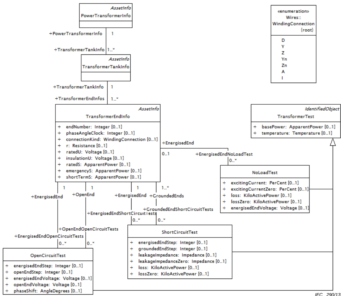
Figure 13 – Modèle de feuilles de données des transformateurs DCIM
