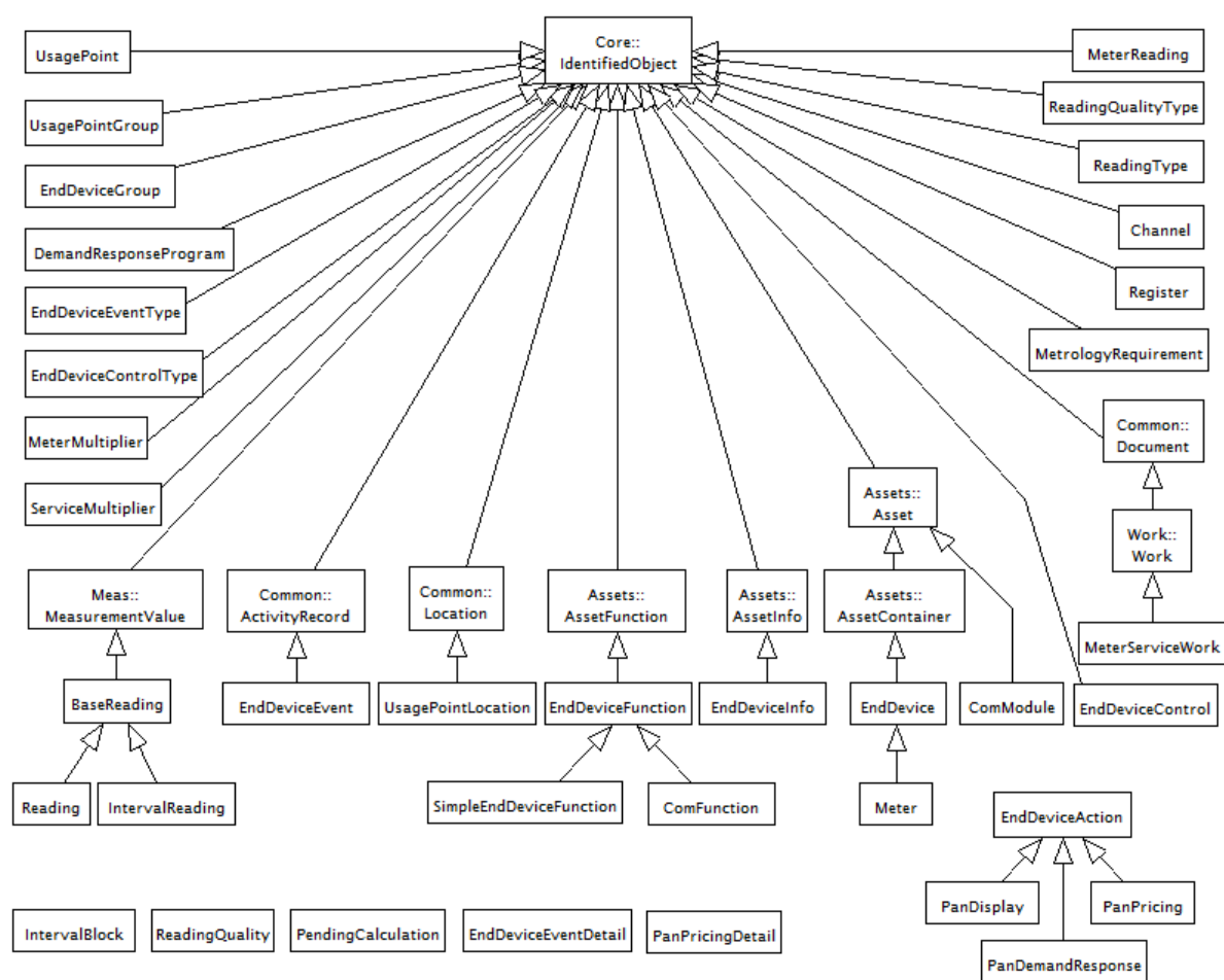
Figure 42 – Diagramme de classe Metering::MeteringInheritance
