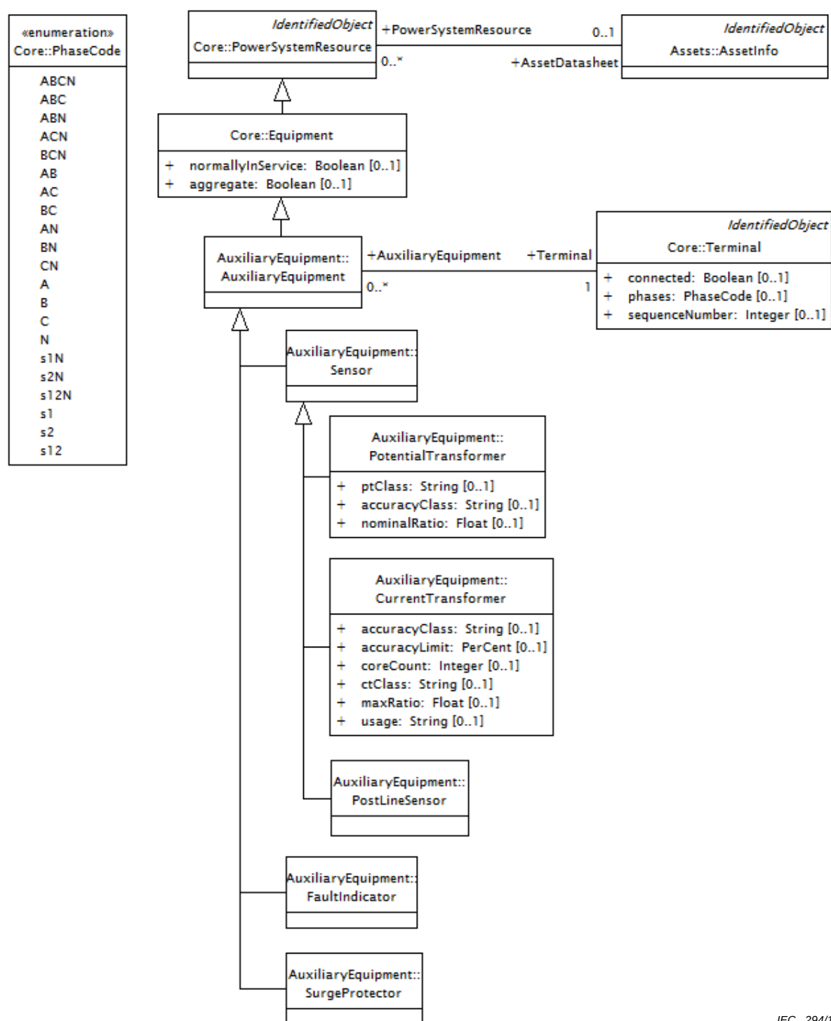
Figure 17 – Équipement auxiliaire DCIM
