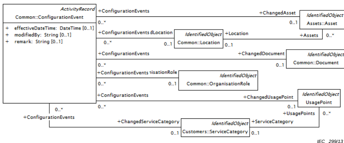
Figure 22 – Événements de configuration pour le comptage
