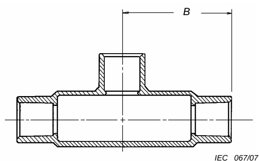
Figure 21 B – (vue de profil)
