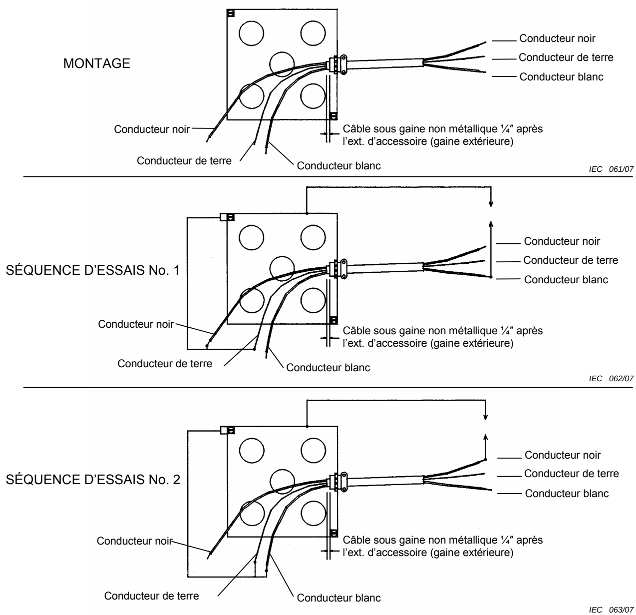
Figure 18 – Montage d'essai pour connecteurs de câbles sous gaine non métallique utilisant un essai diélectrique de 5000 V (9.20.4.2)
