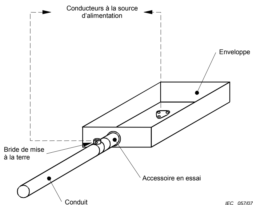
Figure 14 – Essai de courant de défaut utilisant une enveloppe (Paragraphe 9.6.2)
