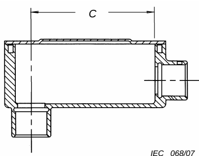
Figure 21 C – Tirage en angle (vue de profil)
