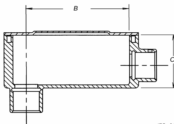
Figure 5b – Tirage en angle (vue latérale)
