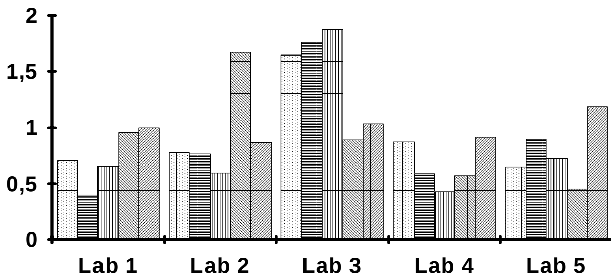
Figure A.1 – Statistiques h de Mandel
