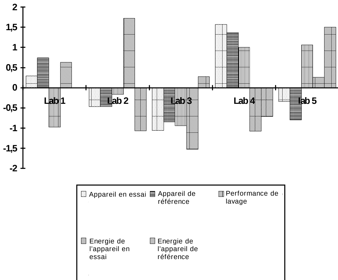
Figure A.1 – Statistiques h de Mandel
