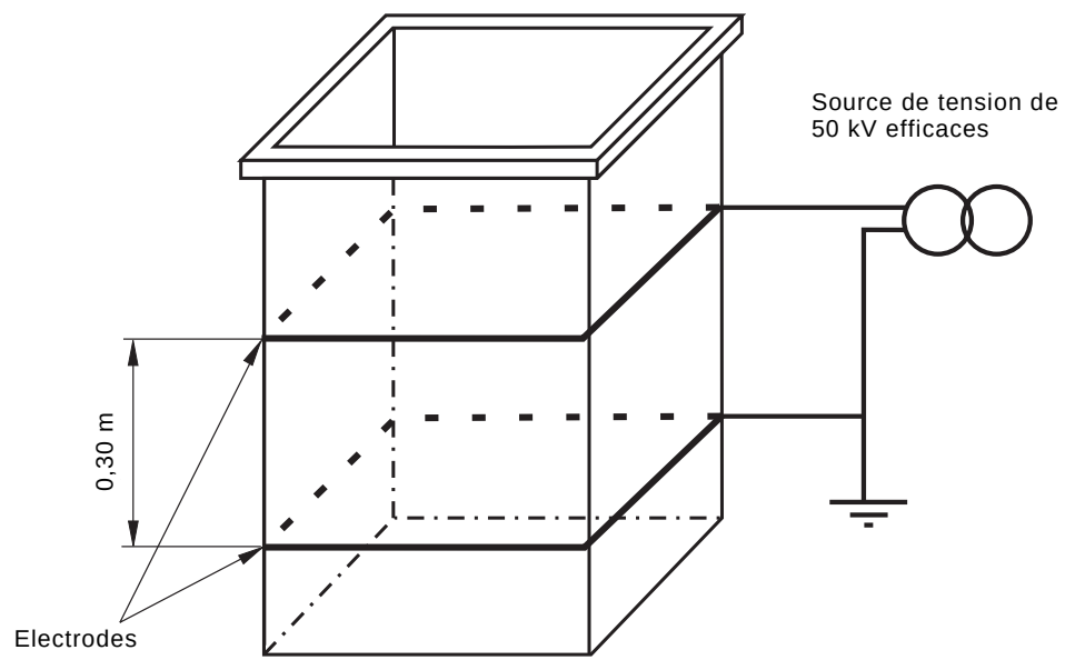
Figure 5 – Essai de surface de la plate-forme ou de la double enveloppe isolante
