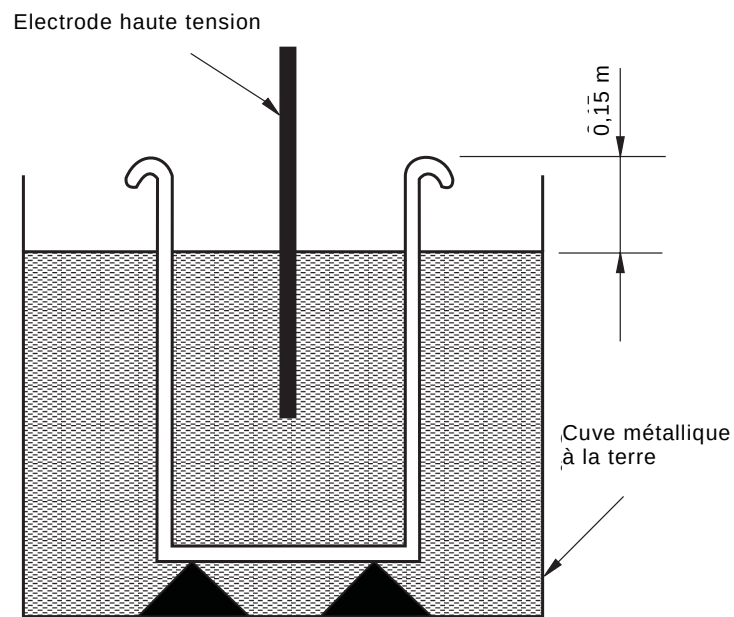
Figure 4 – Essai de perforation de la plate-forme ou de la double enveloppe isolante
