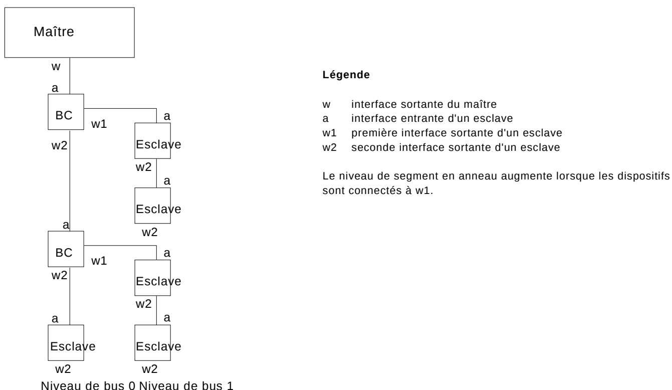
Figure A.1 – Exemple de structure de réseau de Type 8
