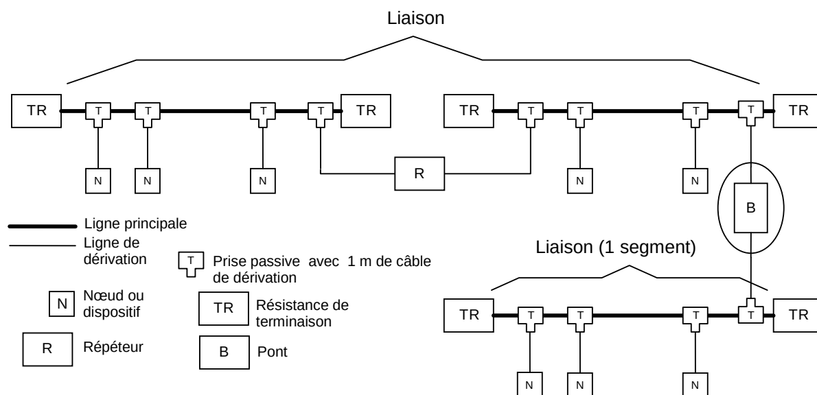
Figure A.9 – Extension du réseau au-delà de 99 nœuds
