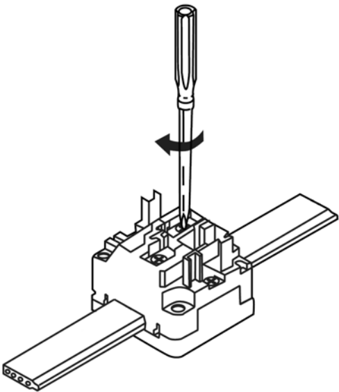
Figure C.37 – Mise en place des contacts IDC dans le câble
