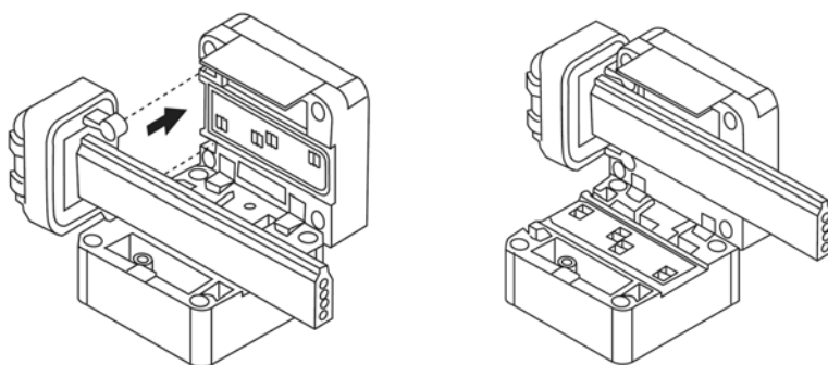
Figure C.40 – Pose de l'embout d'extrémité de l'autre côté du câble
