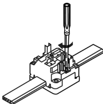
Figure C.36 – Verrouillage de l'ensemble
