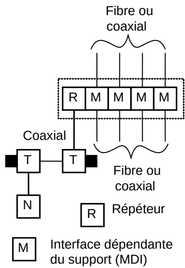
Figure A.7 – Extension d'un réseau au moyen d'une topologie en étoile active
