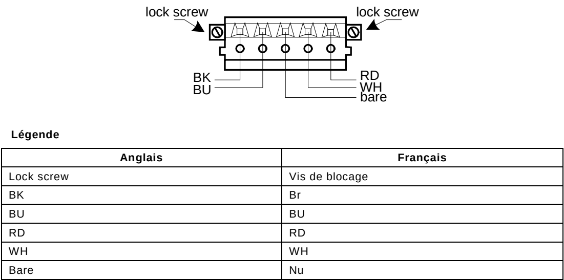
Figure C.9 – Configuration des broches d'un connecteur de type ouvert
