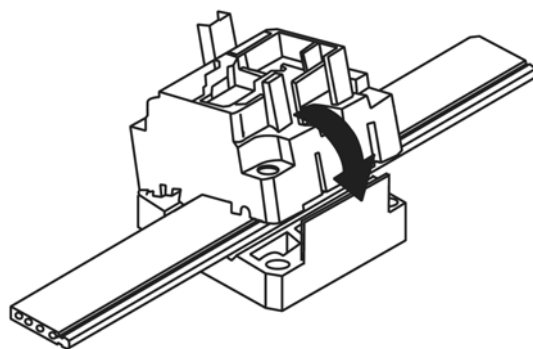
Figure C.34 – Fermeture de l'ensemble
