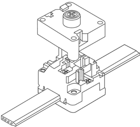
Figure C.42 – Montage des connecteurs
