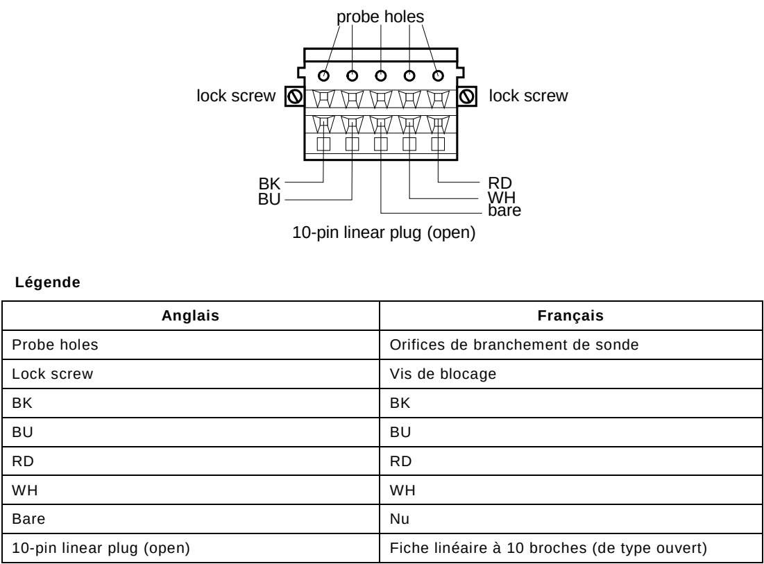
Figure C.10 – Configuration des broches d'un connecteur de type ouvert à 10 positions
