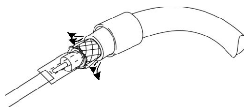
Figure A.37 – Élargissement des blindages
