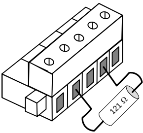
Figure C.48 – Termination de type ouvert
