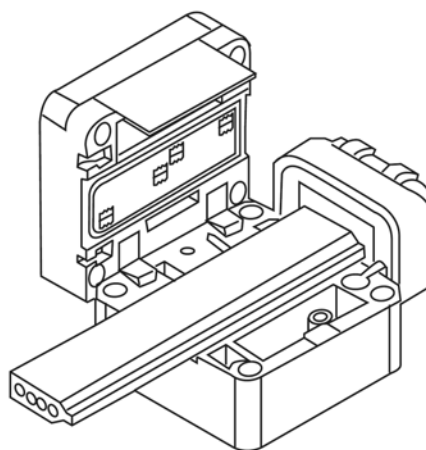
Figure C.39 – Embout d'extrémité positionné
