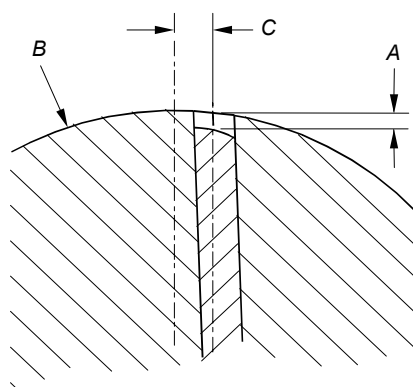
Figure 3 – Dimension de l'interface de la zone de contact de l'extrémité
