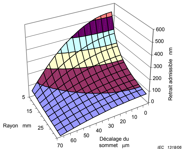
Figure A.1 – Retrait admissible en fonction du rayon d'extrémité et du décalage du sommet – Force de contact minimale de 4,9 N
