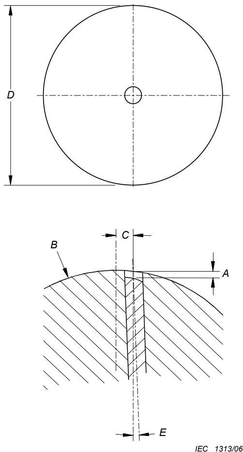
Figure 1 – Dimensions d'interface
