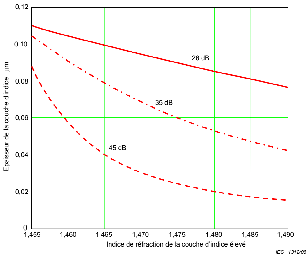
Figure 3 – Indice de réfraction et épaisseur de la couche à indice élevé par rapport à l'affaiblissement de réflexion pour une fibre unimodale typique sans dispersion décalée
