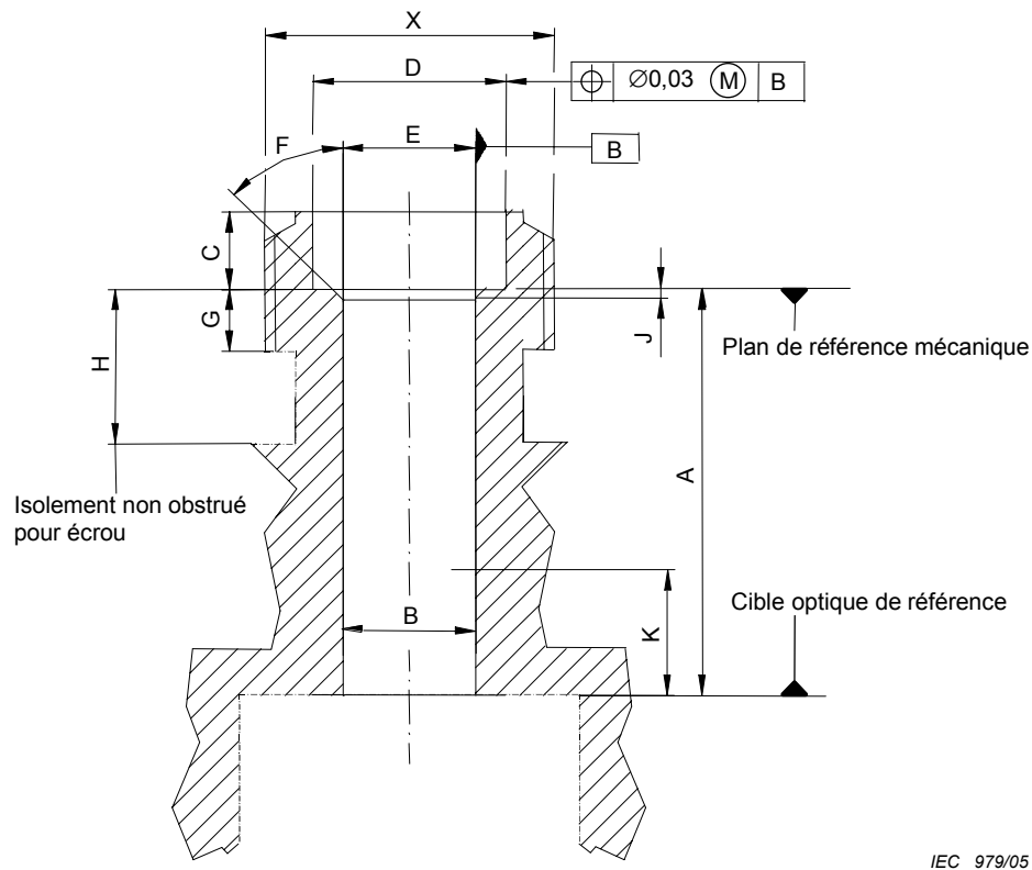
Figure 3 – Interface de connecteurs à prises
