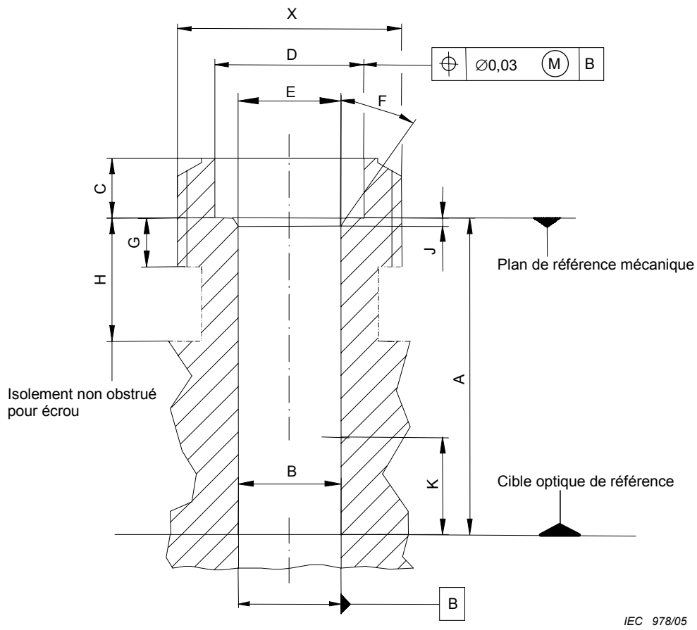
Figure 2 – Interface de connecteurs à adaptateurs
