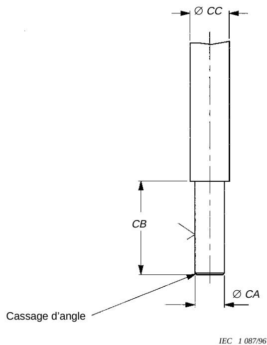
Figure 2b – Calibre pour la bague élastique d'alignement
