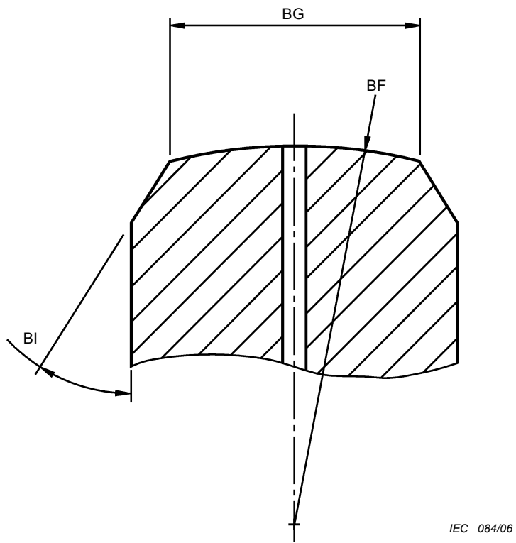
Figure 2 – Interface de connecteur à fiche mâle – Vue agrandie A (voir Tableaux 1 et 2 pour les dimensions)
