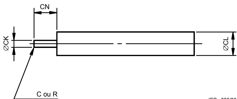
Figure 6 – Pointe de calibrage pour socle à dispositif actif (voir Tableau 7)
