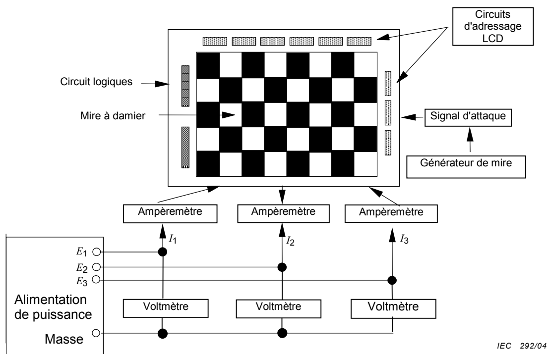
Figure 11 – Exemple de schéma fonctionnel de mesure pour la consommation de courant et d'énergie d'un dispositif à affichage à cristaux liquides
