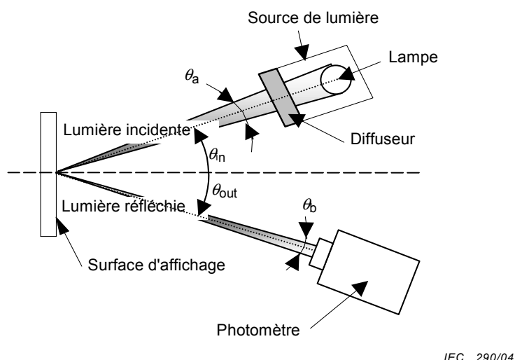
Figure 9 – Exemple de montage normal pour les mesures de réflexion spéculaire
