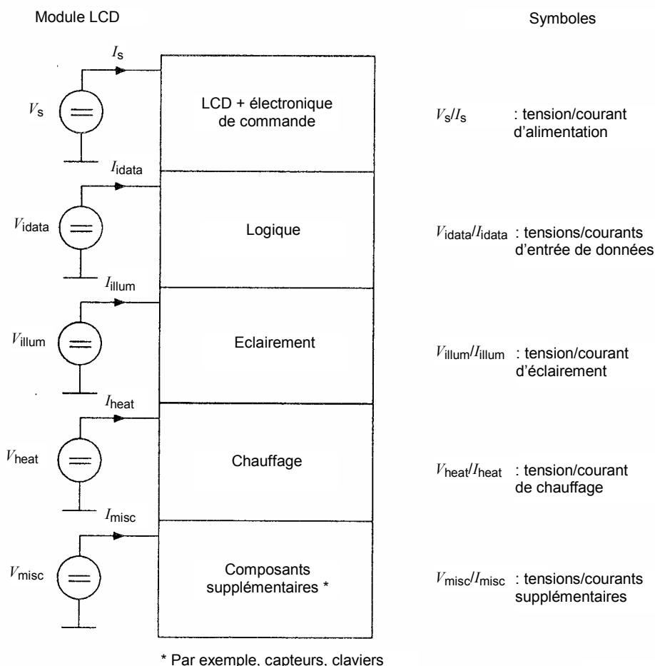
Figure B.6 – Schéma-bloc pour la mesure des courants d'alimentation
