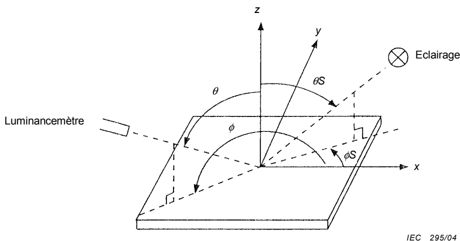
Figure B.3 – Schéma d'un équipement pour le mesurage du rapport de contraste en lumière directionnelle
