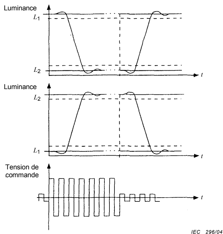
Figure B.4 – Exemples type de réponses dynamiques de deux LCD différents
