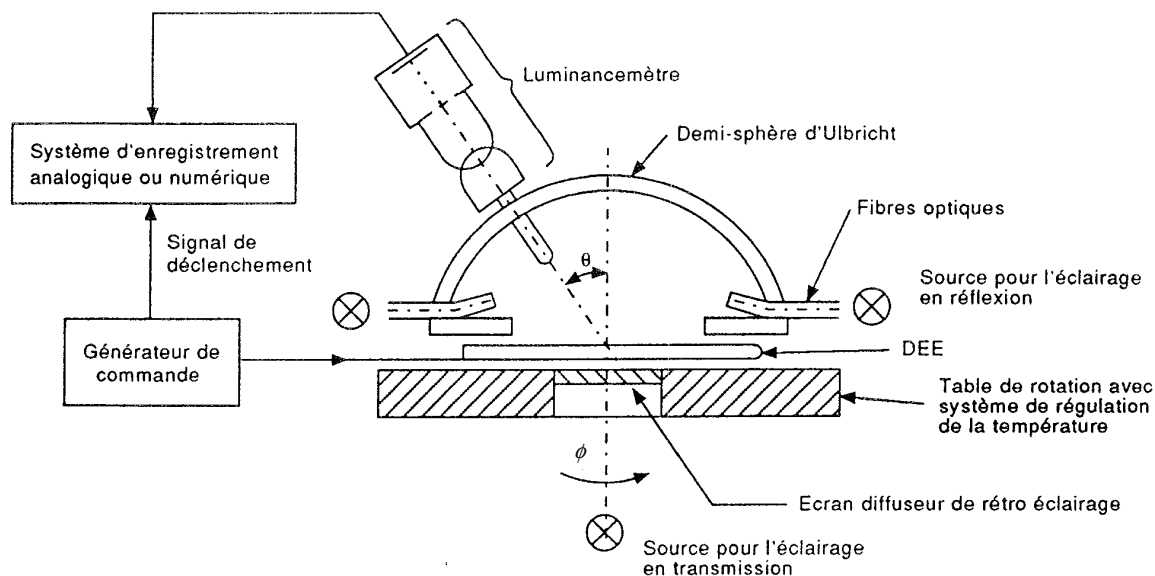
Figure B.2 – Exemple de système pour le mesurage du rapport de contraste en lumière diffuse
