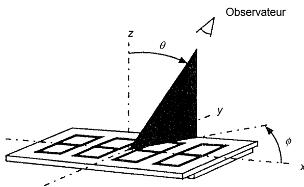
Figure B.1 – Définition de la direction d'observation par l'inclinaison \theta et l'azimut \phi
