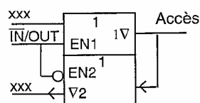
Structure interne d'un accès bidirectionnel
