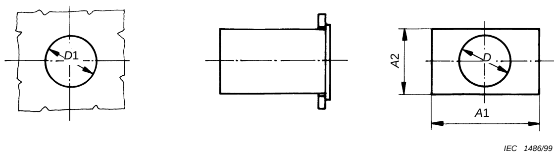
Figure A.2 – Boîtier rond avec cadre rectangulaire
