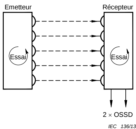
Figure AA.4 – Exemple d'AOPD de type 2 avec essai interne
