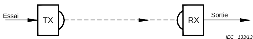
Figure AA.1 – Appareil de détection à simple faisceau
