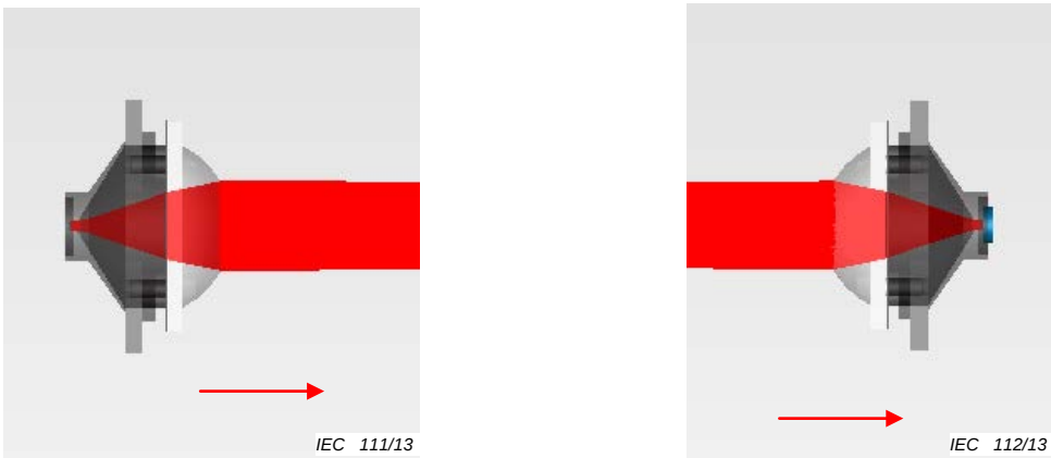
Figure 12 – Exemple de sous-système optique: Emetteur à gauche – Récepteur à droite
