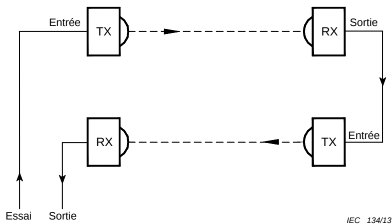
Figure AA.2 – Montage en série des dispositifs de détection à simple faisceau
