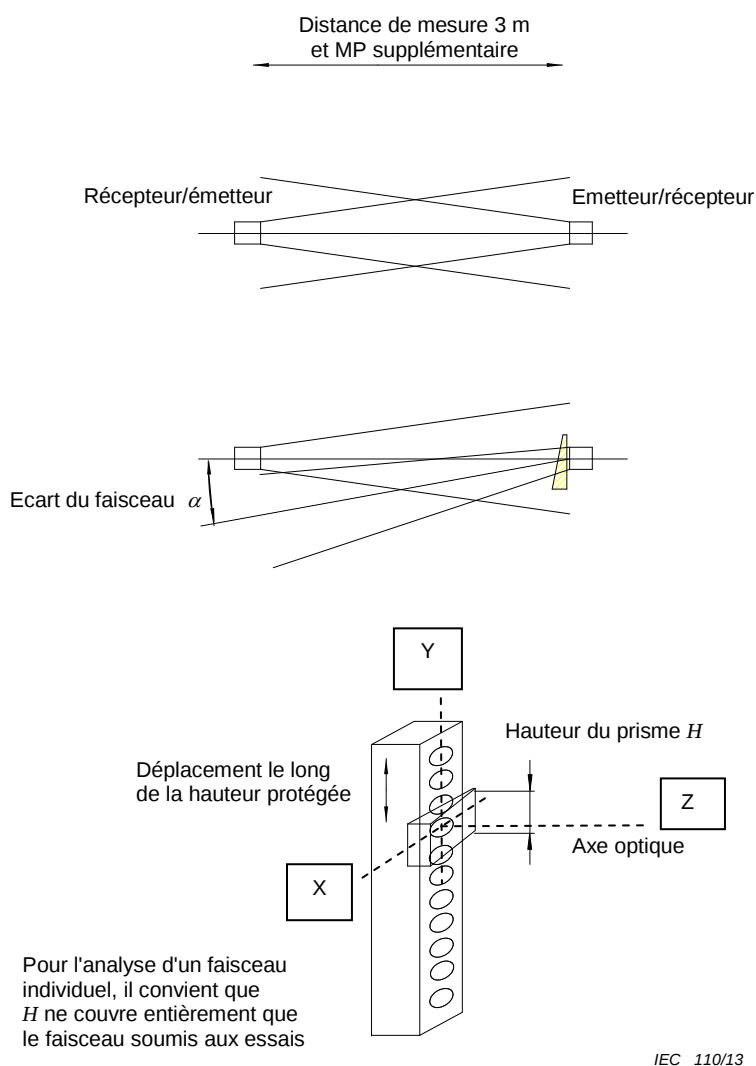
Figure 10 – Essai de l'EEA à l'aide du prisme
