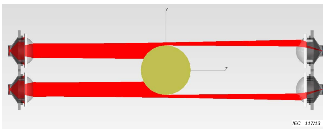
Figure 17 – Exemple d'éprouvette d'essai dans le modèle du sous-système optique avec un rayonnement traversant sur le récepteur
