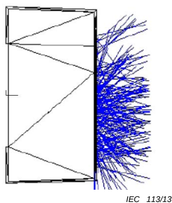
Figure 13 – Exemple de modèle de LED CMS
