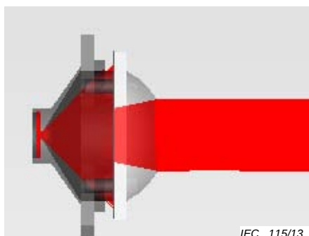
Figure 15 – Exemple de modèle d'émetteur avec faisceaux verrouillés en interne par diaphragme
