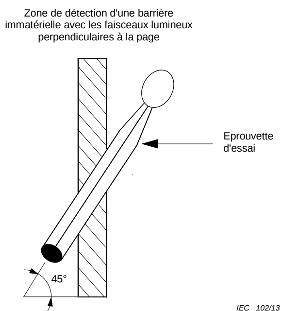
Figure 3 – Epreuve d'essai inclinée à 45°
