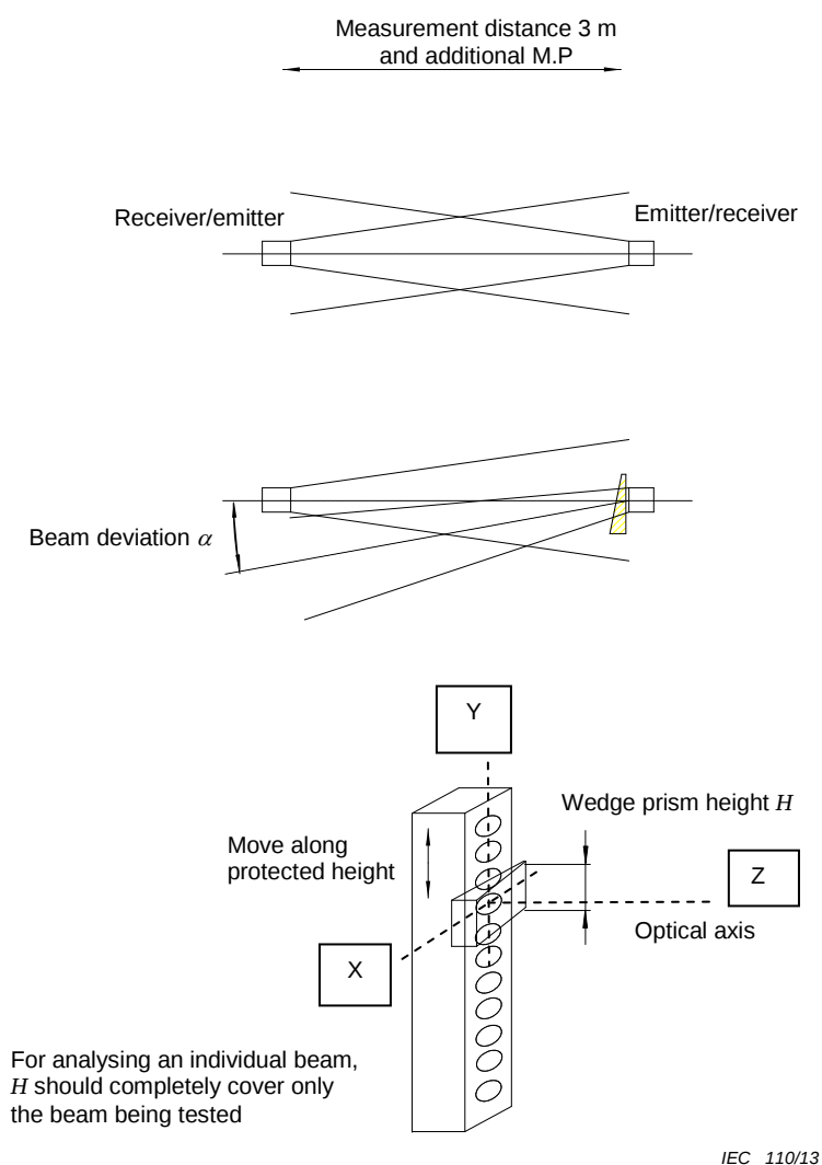
Figure 10 – EAA test using prism
