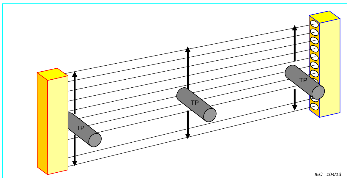
Figure 4 – Epreuve d'essai inclinée à 90°
