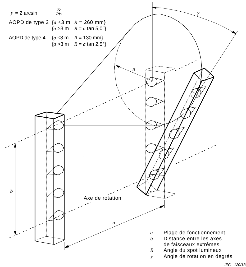
Figure 20 – Essai de désalignement de l'AOPD
