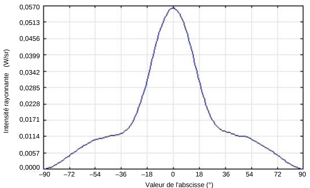
Figure 14 – Exemple de distribution d'intensité d'un émetteur
