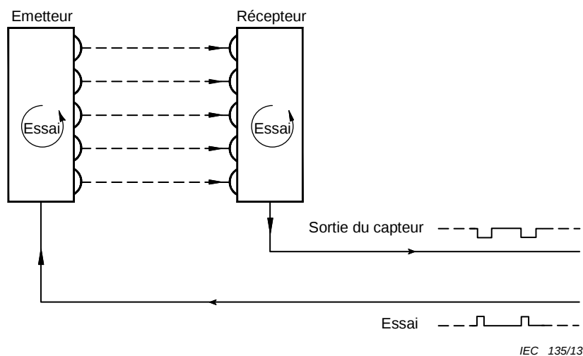
Figure AA.3 – Ensemble de faisceaux multiples testés individuellement
