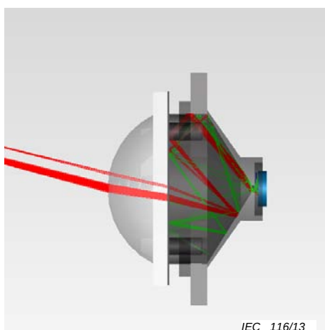
Figure 16 – Exemple d'unité de réception avec une partie du faisceau en dehors de l'axe réfléchi à l'intérieur sur les éléments mécaniques
