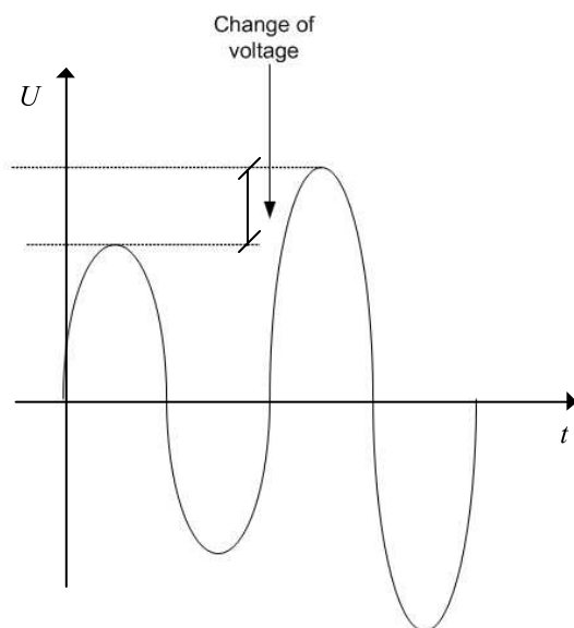
Figure 17 – Variation brusque de tension avec tension d'alimentation en courant continu
