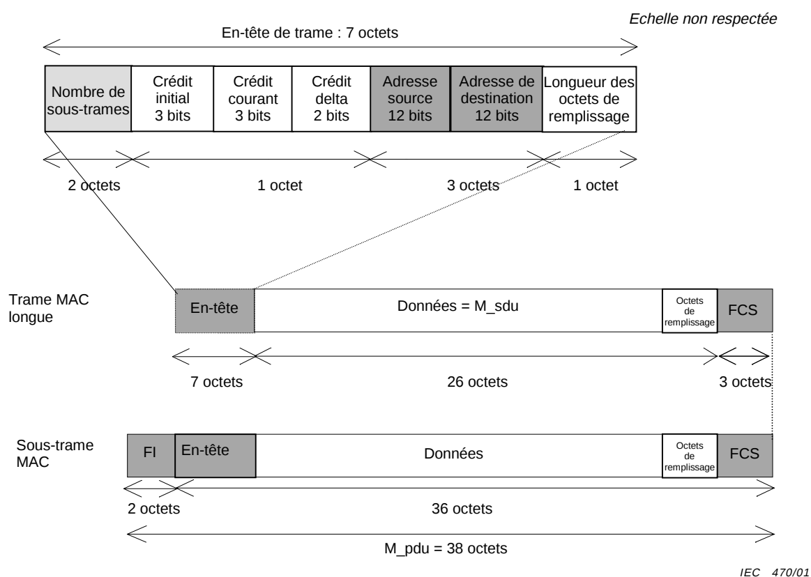
Figure 8 – Trame MAC longue constituée d'une seule sous-trame
